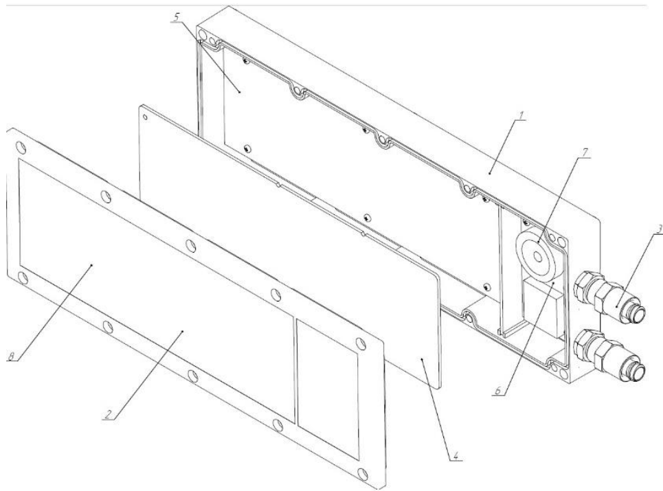
1-Корпус; 2-крышка; 3-кабельные вводы; 4-трафарет; 5-отсек подсветки; 6-коммутационный отсек; 7-зуммер; 8-светопропускающее окно.
