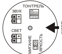
Рис.4 - Расположение клеммников и микропереключателей в коммутационном отсеке оповещателя «Плазма»П- СЗ
