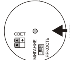
Рис.5 - Расположение клеммников и микропереключателей в коммутационном отсеке оповещателя «Плазма»П - С
