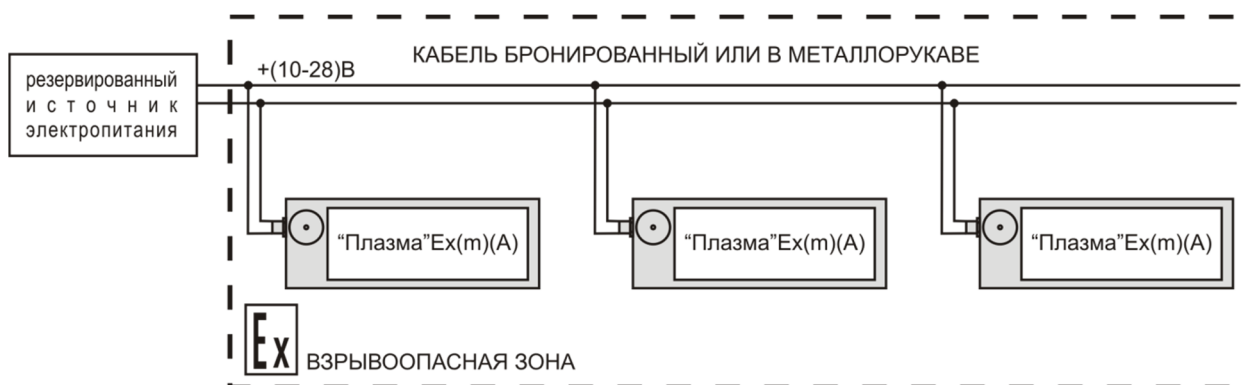
Рис.9 Подключение «Плазма»Ex(m)(A) 2ExmIT6 X/ РПExmI X к линии питания 10-28 В постоянного тока. Линия прокладывается бронированным кабелем или кабелем в металлорукаве.
