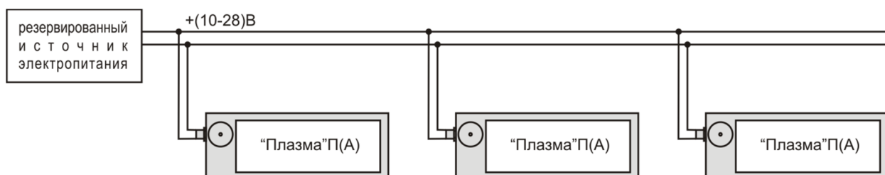
Рис.8 Подключение «Плазма»П(А) к линии питания 10-28 В постоянного тока.
