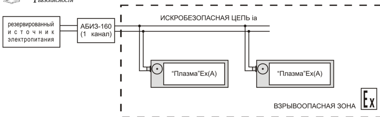
Рис.10 Подключение «Плазма»Ex(A) 0ExiaICT6 X / POExiaI X к линии питания 12 В постоянного тока искробезопасной цепи ia. На один канал искрозащитного барьера АБИЗ-160 можно подключить один «Плазма»Ex(A) с включённым микропереключателем «ЯРКО» или два «Плазма»Ex(A) с выключённым микропереключателем «ЯРКО».
