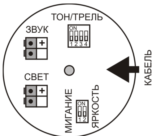
Рис.4 Расположение клеммников и микропереключателей в коммутационном отсеке оповещателей «Плазма»Ех,Ех(м),П – СЗ
