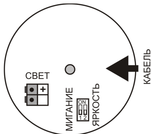
Рис.5 Расположение клеммников и микропереключателей в коммутационном отсеке оповещателей «Плазма»Ех,Ех(м),П - С
