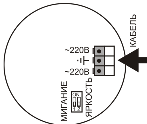
Рис.7 Расположение клеммников и микропереключателей в коммутационном отсеке оповещателей «Плазма»П220 - С
