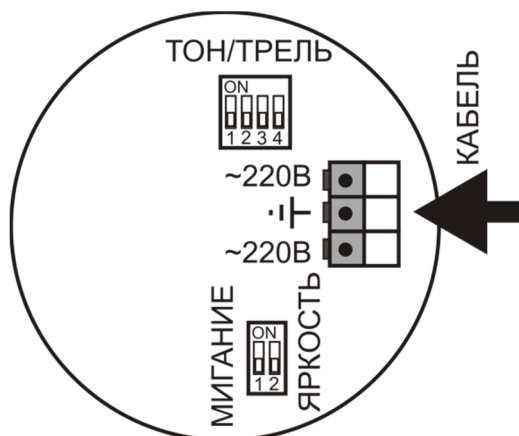
Рис.6 Расположение клеммников и микропереключателей в коммутационном отсеке оповещателей «Плазма»П220 - СЗ
