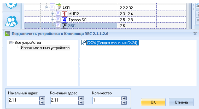
Рисунок 5.20 – Подключение «Ключница ЭВС»
