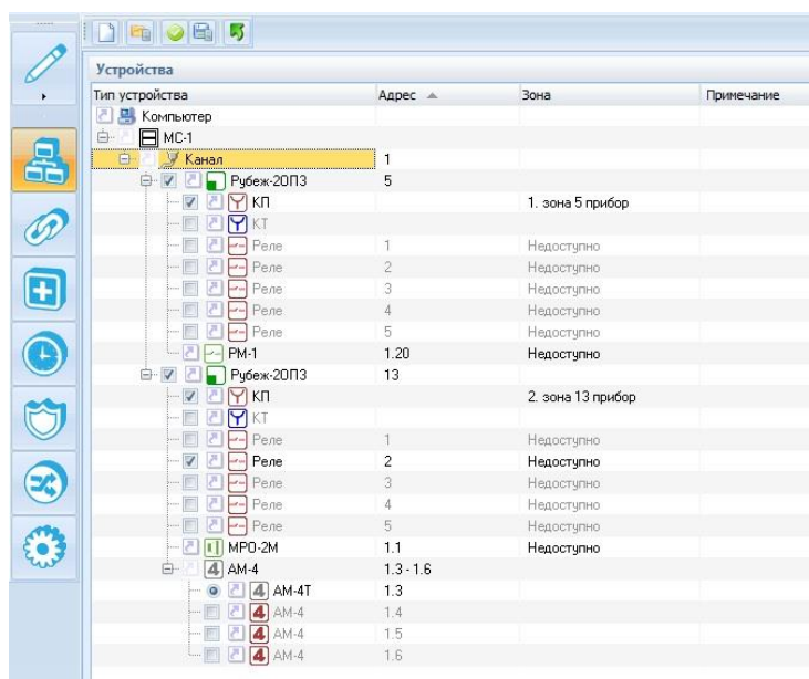
Рисунок Б.1 – В дерево устройств подключены два прибора «Рубеж-2ОП» прот. R3
