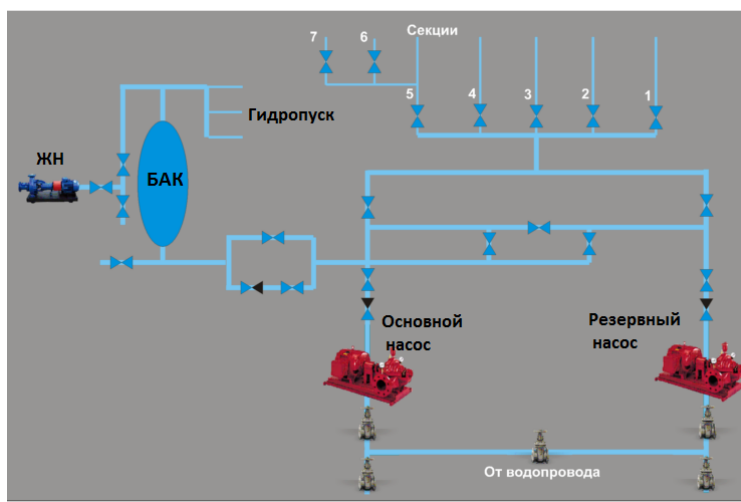
Рисунок Г.1 – Графическая схема насосной станции, используемой на объекте
