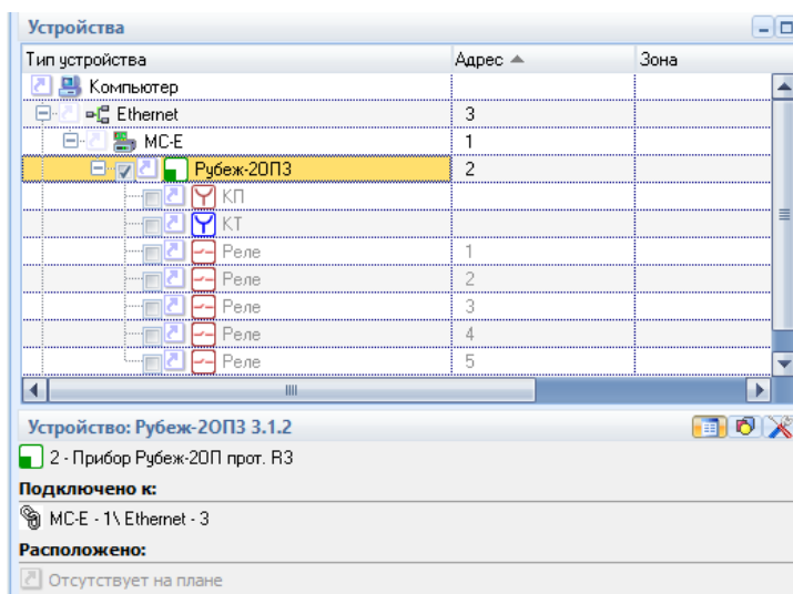
Рисунок 5.43 – Подключение «Рубеж-2ОП» прот. R3 к компьютеру через МС-Е
