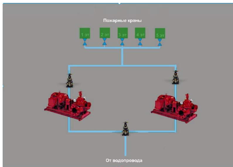
Рисунок Г.25 – Система внутреннего пожаротушения
