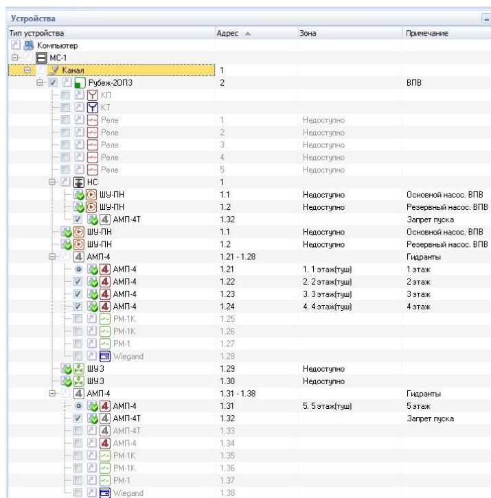
Рисунок Г.27 – Дерево устройств системы
