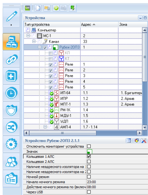
Рисунок 2.2 – Выбор топологии АЛС прибора «Рубеж-2ОП» прот. R3
