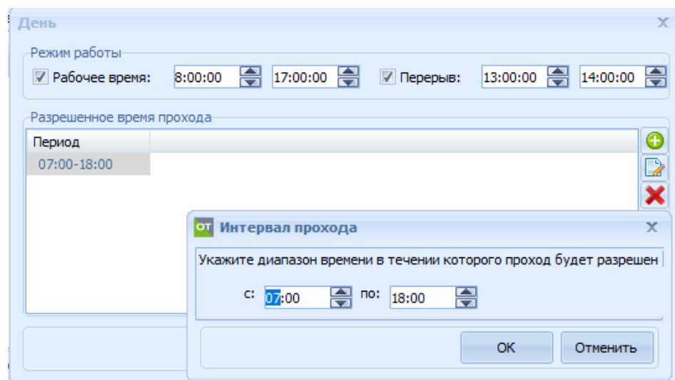
Рисунок 25.18 – Окно «День»
