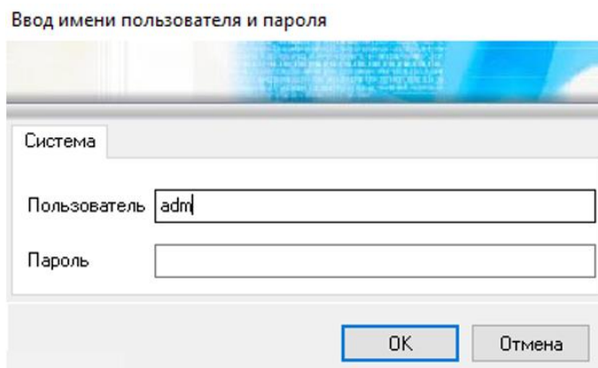
Рисунок 18.1 – Окно авторизации
