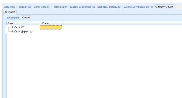
Рисунок 33.4 –Вкладка Ключи
