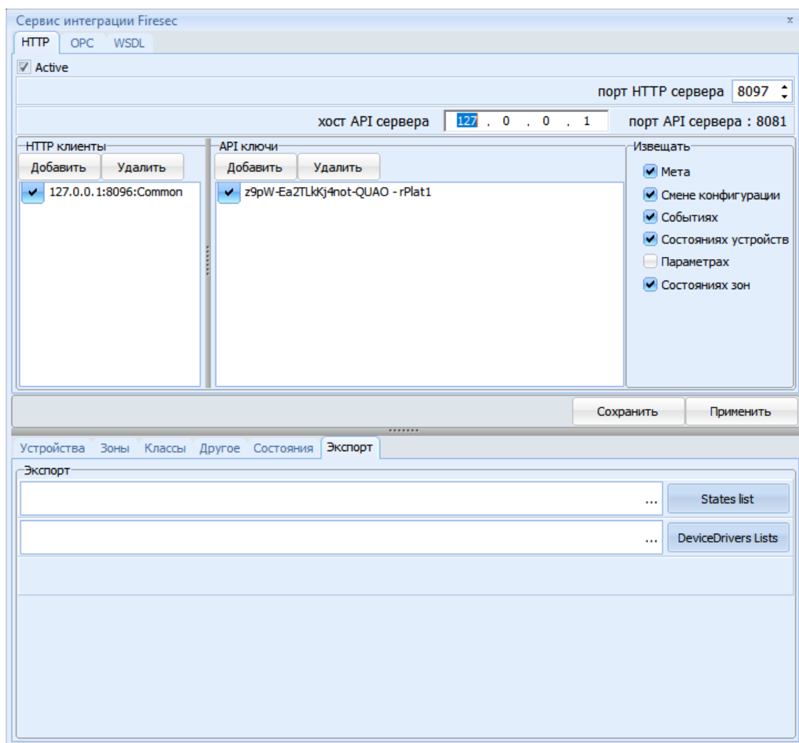
Рисунок 29.6 – Вкладка экспорт
