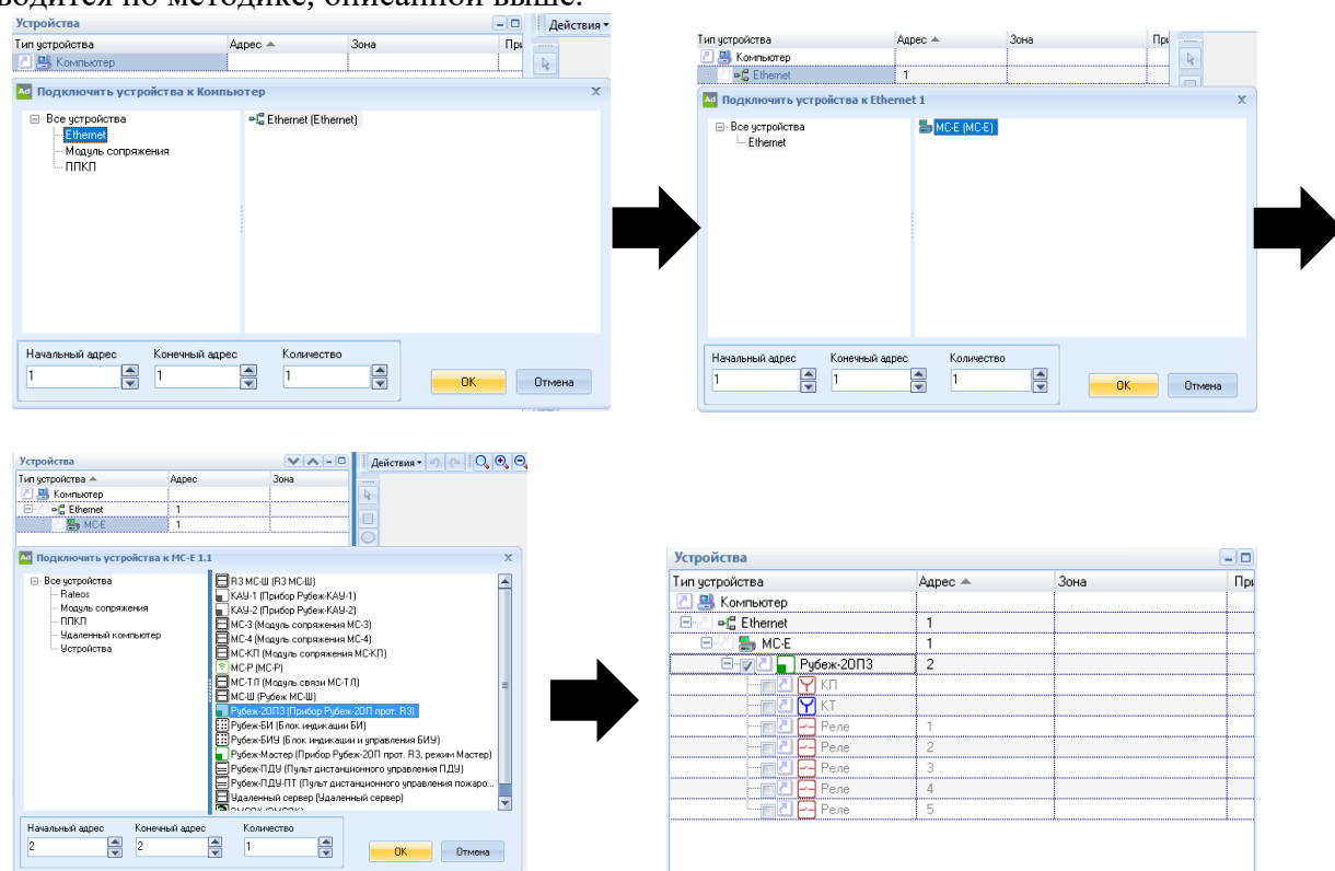
Рисунок 5.5.2 – Подключение «Рубеж-20П» прот. R3 к компьютеру по Ethernet
