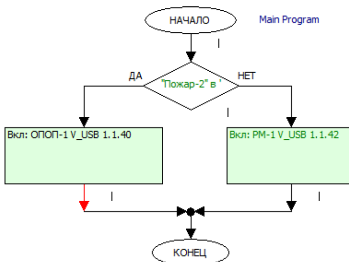
Рисунок 9.19 – Пример простой блок схемы
