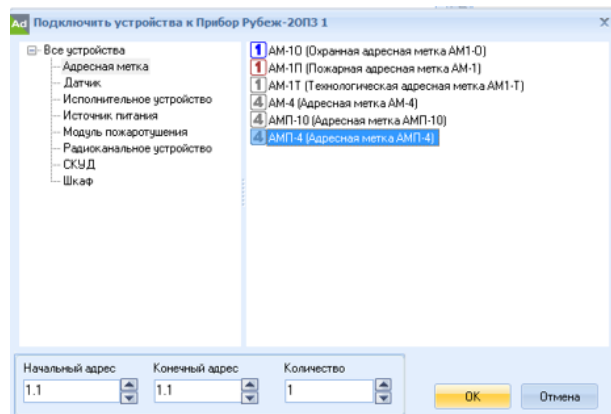
Рисунок В.4 – Подключение к «Рубеж-20П» прот.Р3 адресной метки АМП-4
