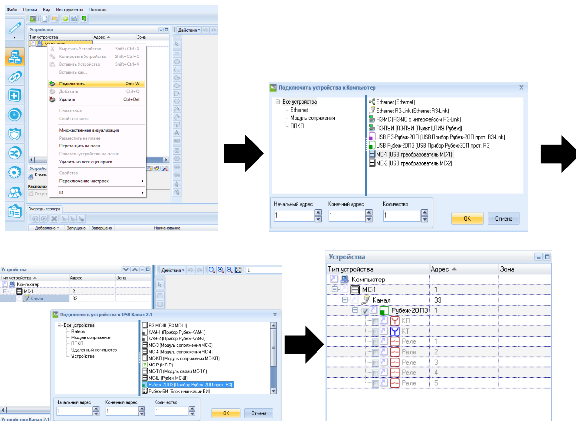
Рисунок 5.5.1 – Подключение ППКП через модуль сопряжения MC-1
