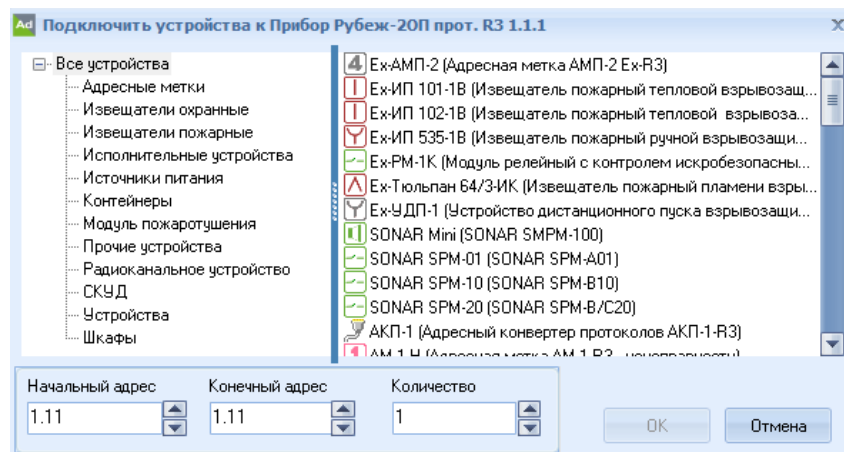
Рисунок А.2 – Подключение МКД-2 к «Рубеж-20П» прот. R3
