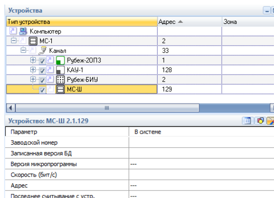
Рисунок 5.28 – Пример подключения МС-Ш в дереве устройств
