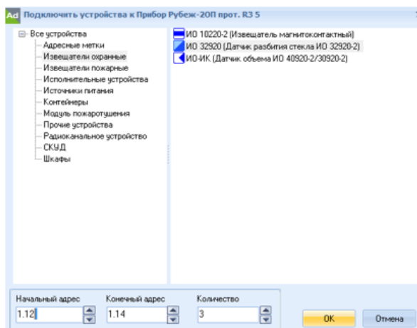
Рисунок В.6 – Подключение к «Рубеж-20П» прот. R3 трех датчиков ИО 32920-2
