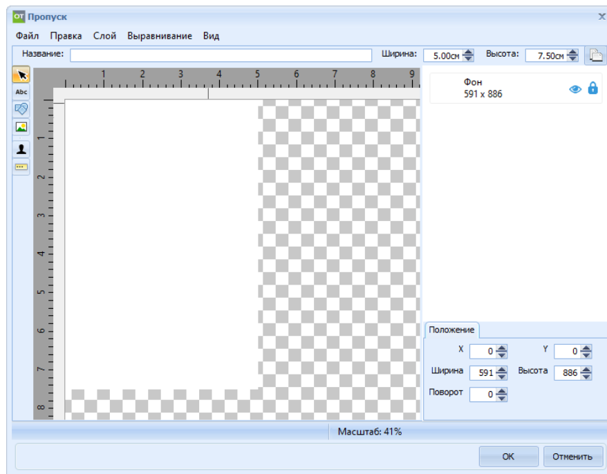
Рисунок 25.24 – Окно Пропуск
