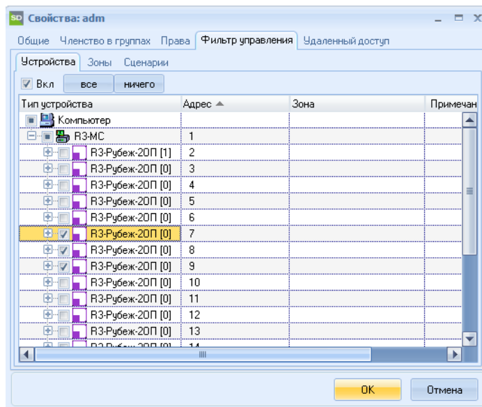
Рисунок 3.17 – «Фильтр управления»
