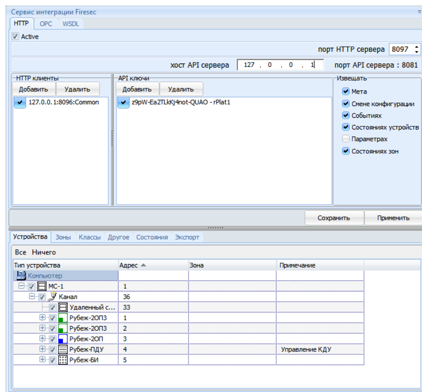
Рисунок 29.2 – Окно «IntegrationClient»
