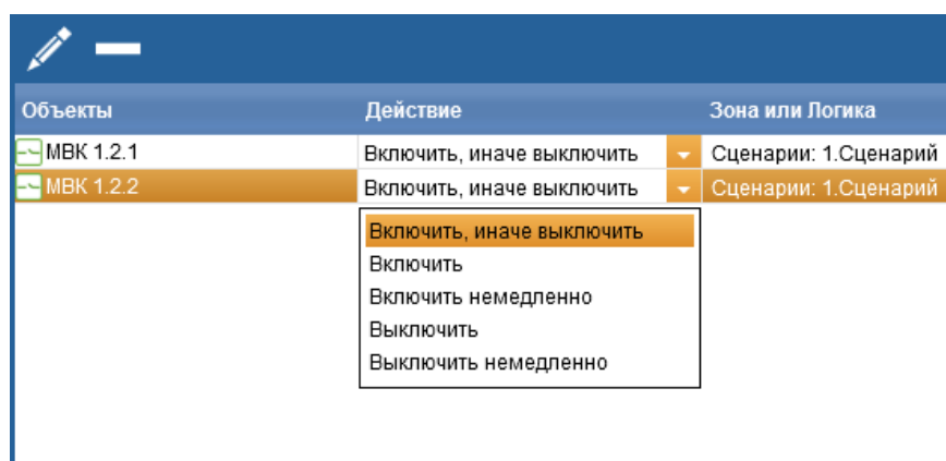
Рисунок 5.15 – Настройка параметров работы исполнительного устройства
