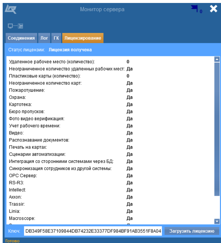
Рисунок 1.12 – Окно Монитор сервера приложений Глобал, вкладка Лицензирование
