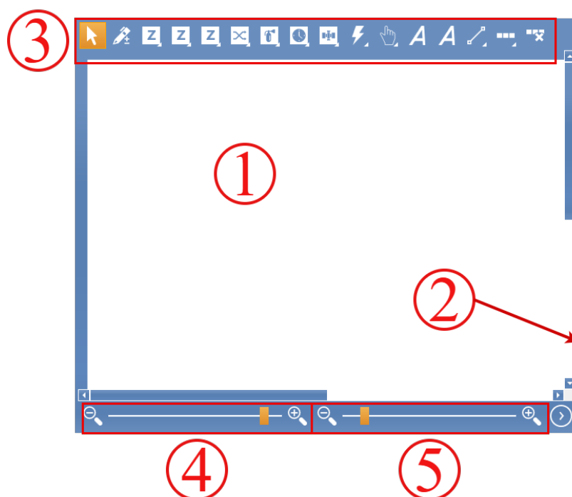
Рисунок 4.7 – Рабочая область в окне Планы
