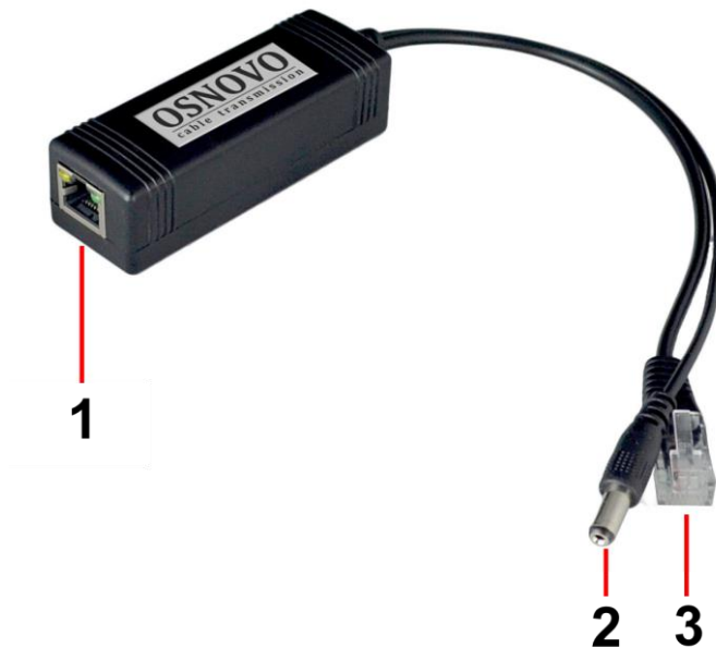
Рис. 2 PoE Splitter/3, разъемы и индикаторы
