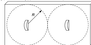
Рис.2 Основная защита, R = 2м., защищаемая площадь > 75%
