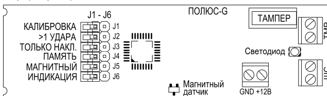
Рис.1 Плата извещателя
