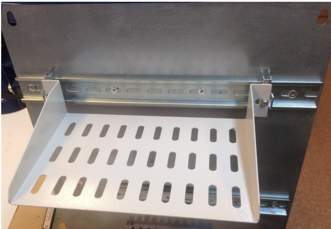
Рис.1-1 Установка полки для оборудования на din-рейку монтажной панели.
