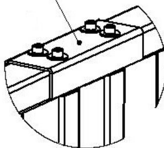
рис. 3 Установка накладки PERCo-RF01 0-05
