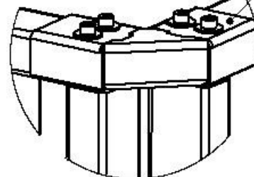
рис. 2 Установка накладки PERCo-RF01 0-04
