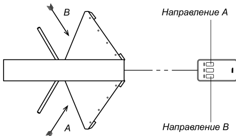
Рисунок 8. Стандартная ориентация ПДУ относительно стойки турникета
