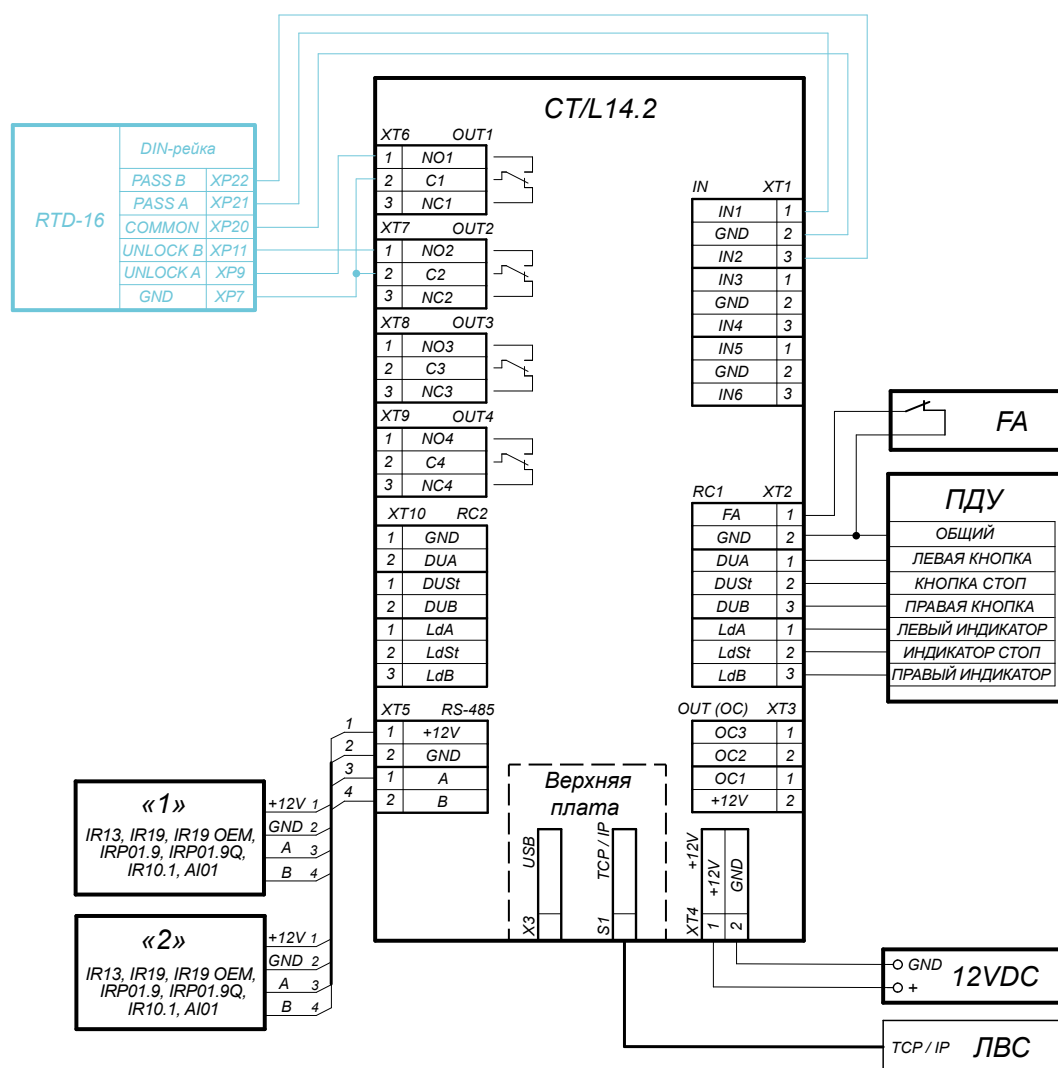
Схема подключения турникета к контроллеру СКУД (на примере контроллера СТ/L14.2)
