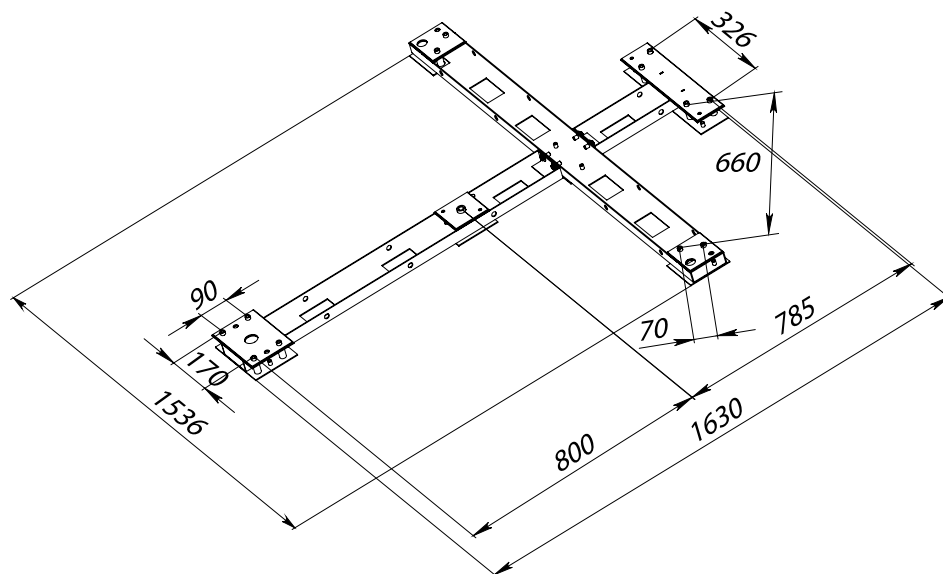
Установка рамы
