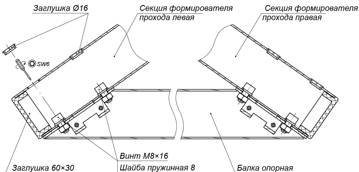
Рисунок 12. Крепление балки опорной (7) к секциям (6) формователя прохода
