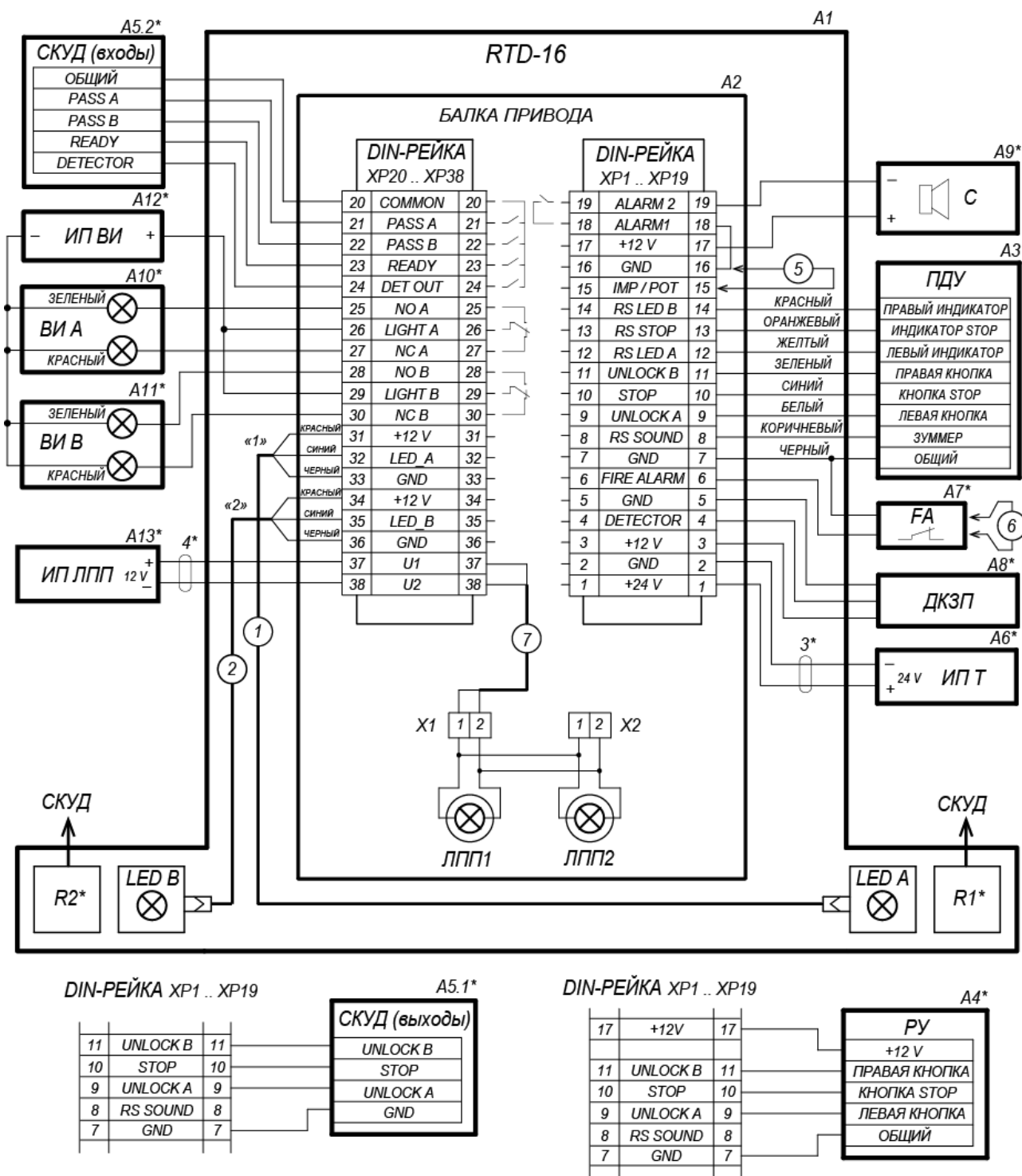
Рисунок 21. Схема подключения турникета и дополнительного оборудования 1
