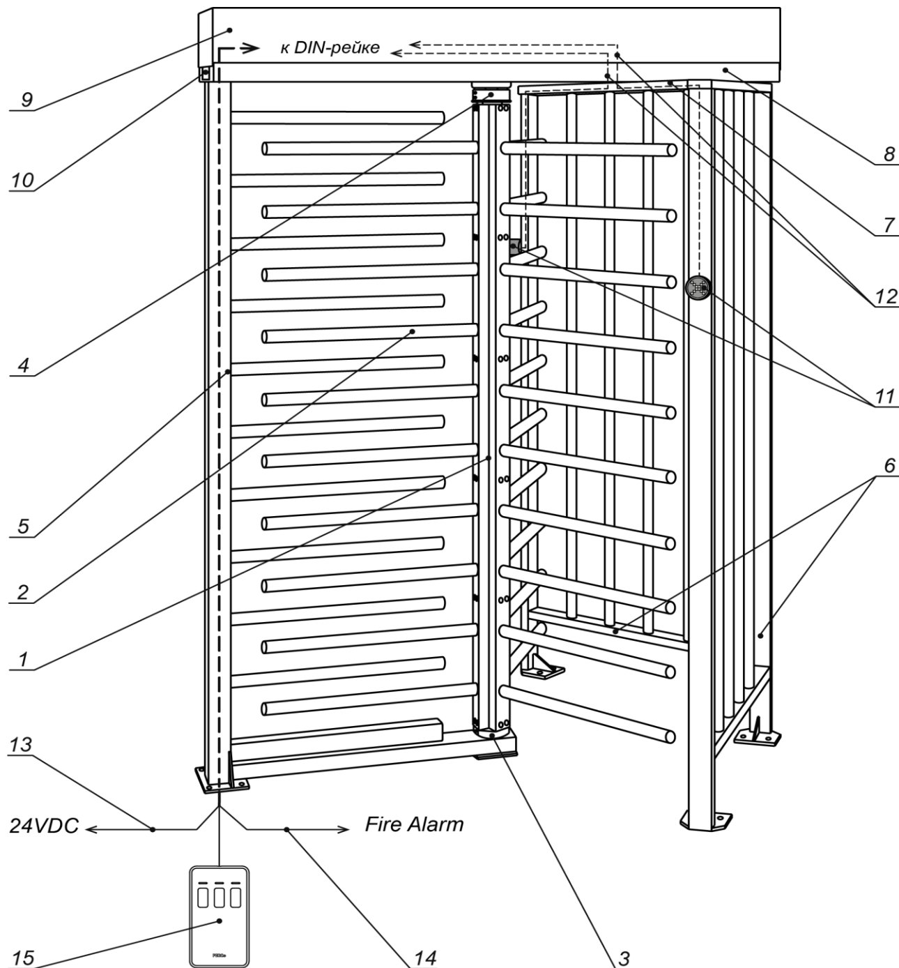
Рисунок 2. Устройство турникета:
