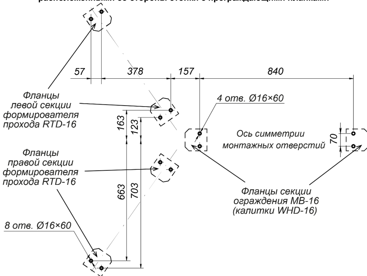
Рисунок 28. Схема разметки для монтажа турникета с ограждением или калиткой, расположенными со стороны секций формирователя прохода 2
