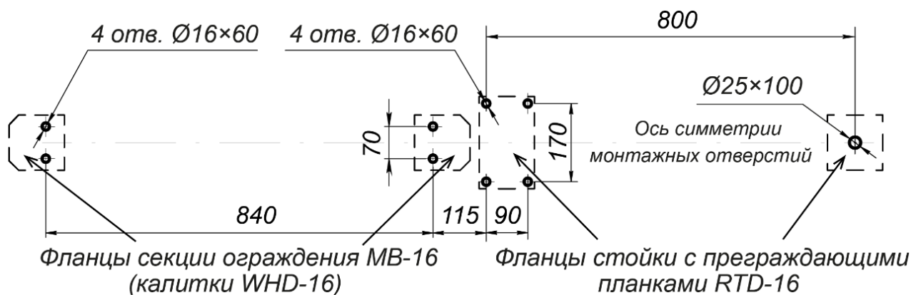
Рисунок 27. Схема разметки для монтажа турникета с ограждением или калиткой, расположенными со стороны стойки с преграждающими планками 1
