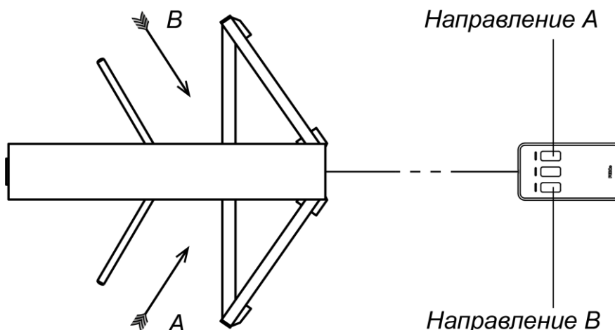
Рисунок 6. Стандартная ориентация ПДУ относительно стойки турникета
