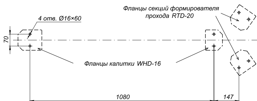
Схема разметки отверстий для совместного монтажа турникета и калитки WHD-16
