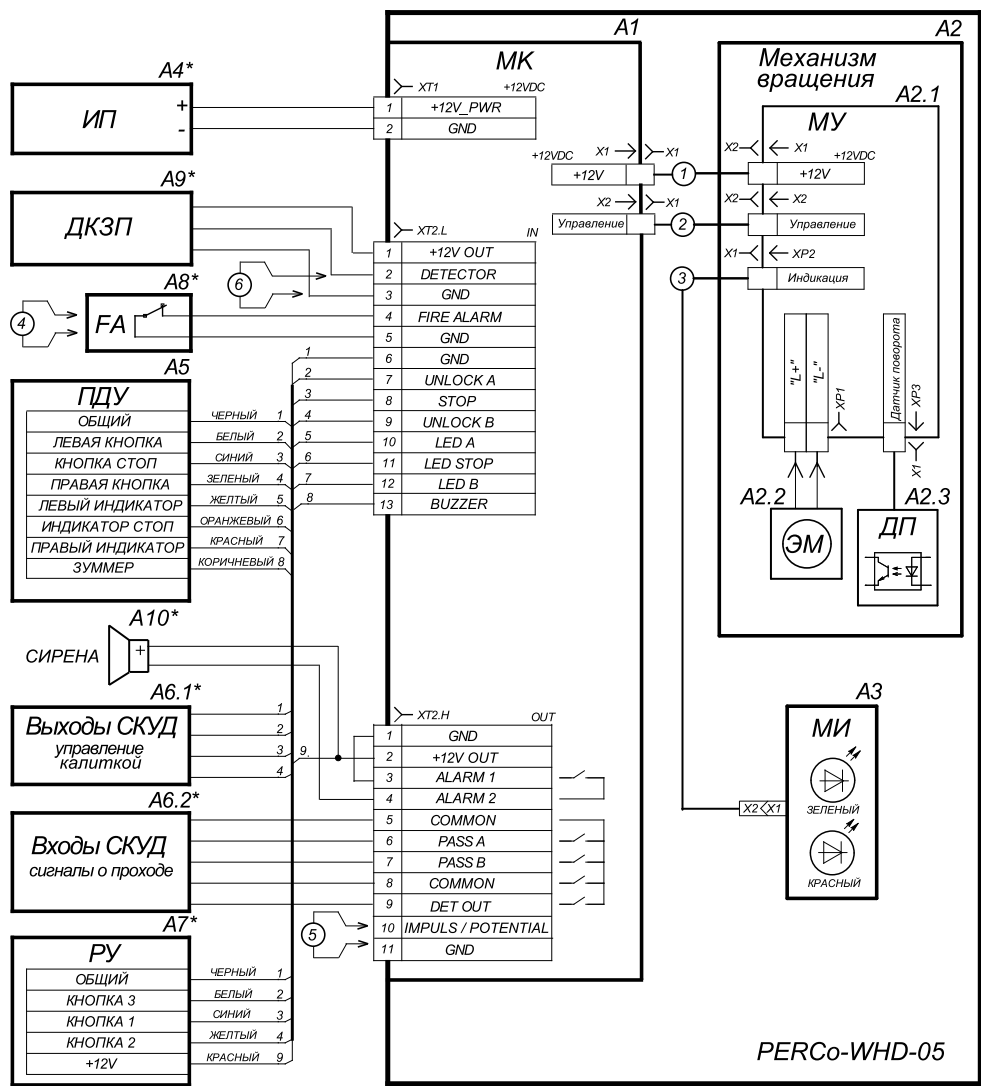
Схема подключения калитки WHD-05
