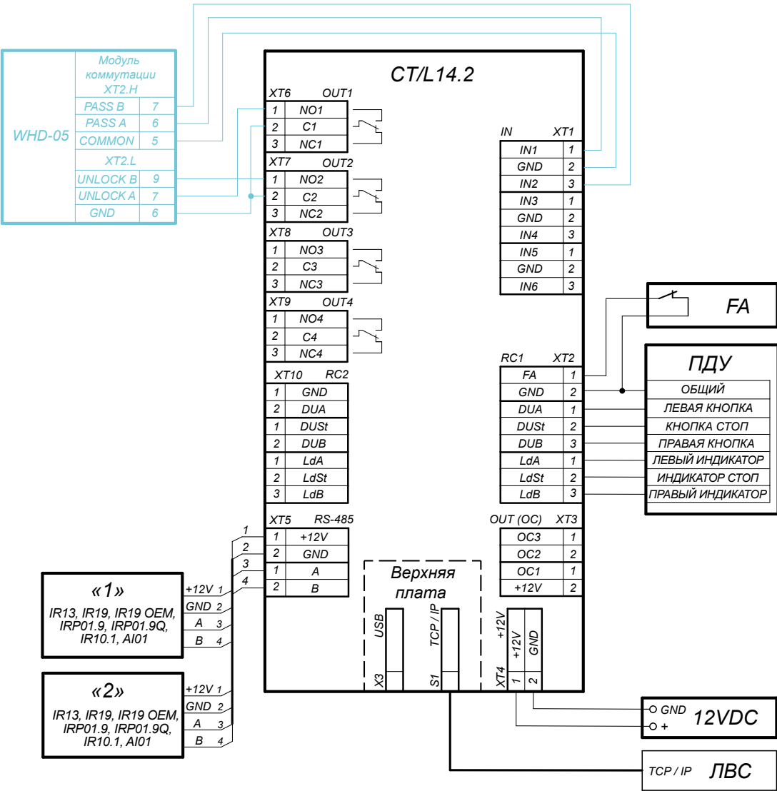
Пример схемы подключения калитки к контроллеру СКУД
