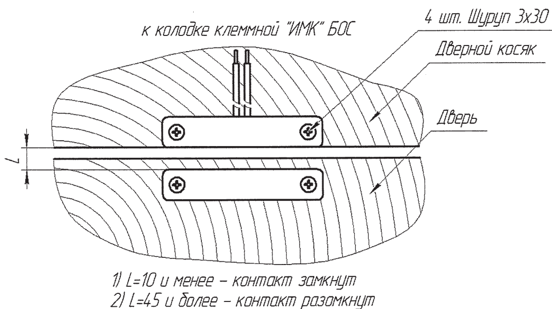
Рисунок 2.3 – Пример установки ИМК на двери
