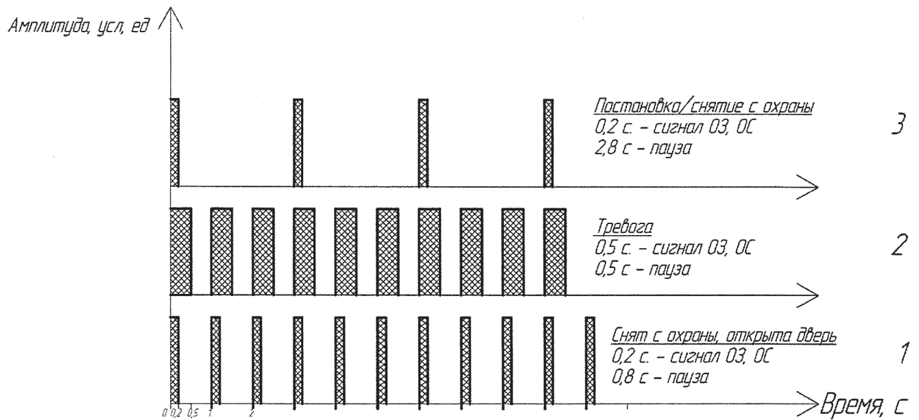
Рисунок В.3 – Временные интервалы ОС и ОЗ
