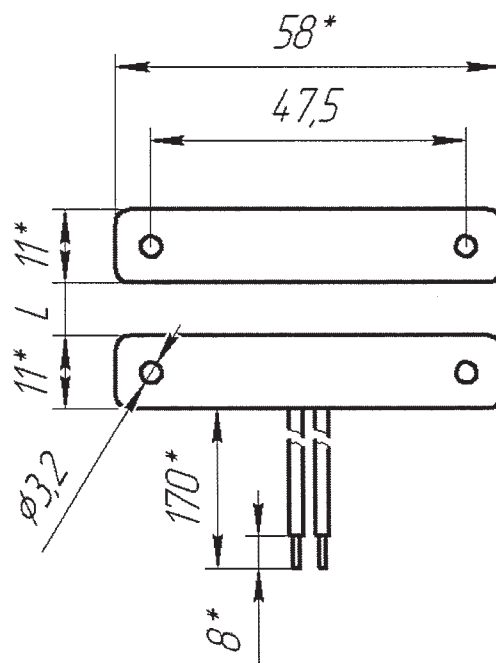
Рисунок 2.2 – Крепление ИМК
