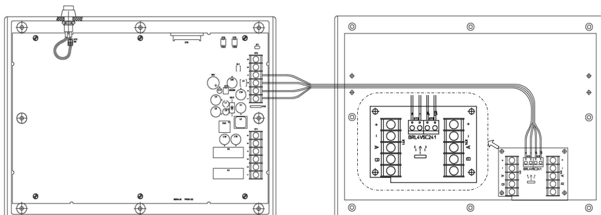
Рис. 3 Схема подключения ППД-01
