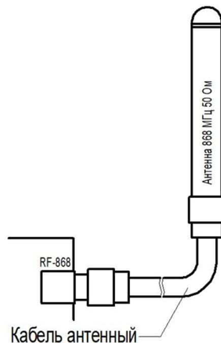
Рисунок 6 - Подключение антенны
