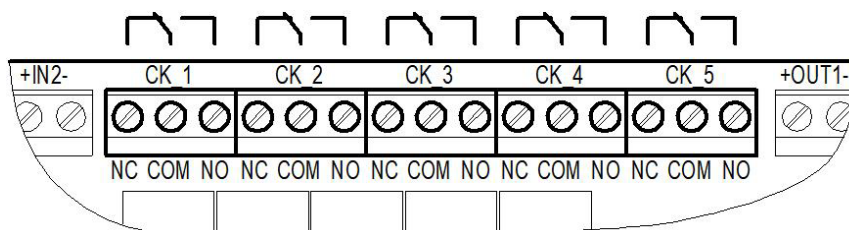
Рисунок 17 - Схема подключения к СК ППК
