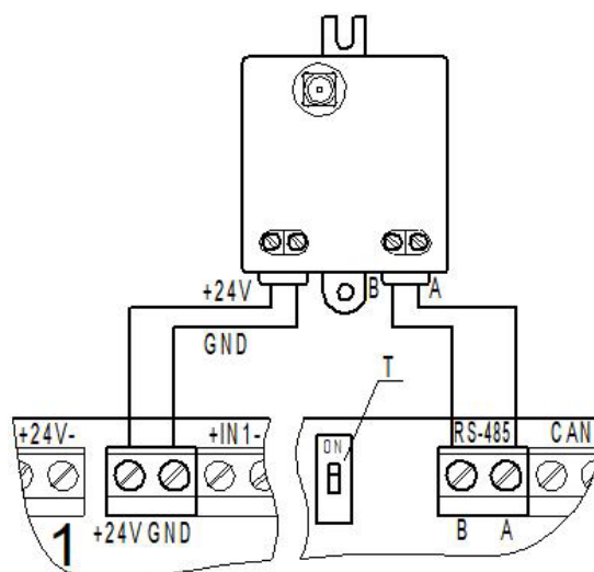
Т – переключатель оконечного резистора (терминатора) интерфейса RS-485
