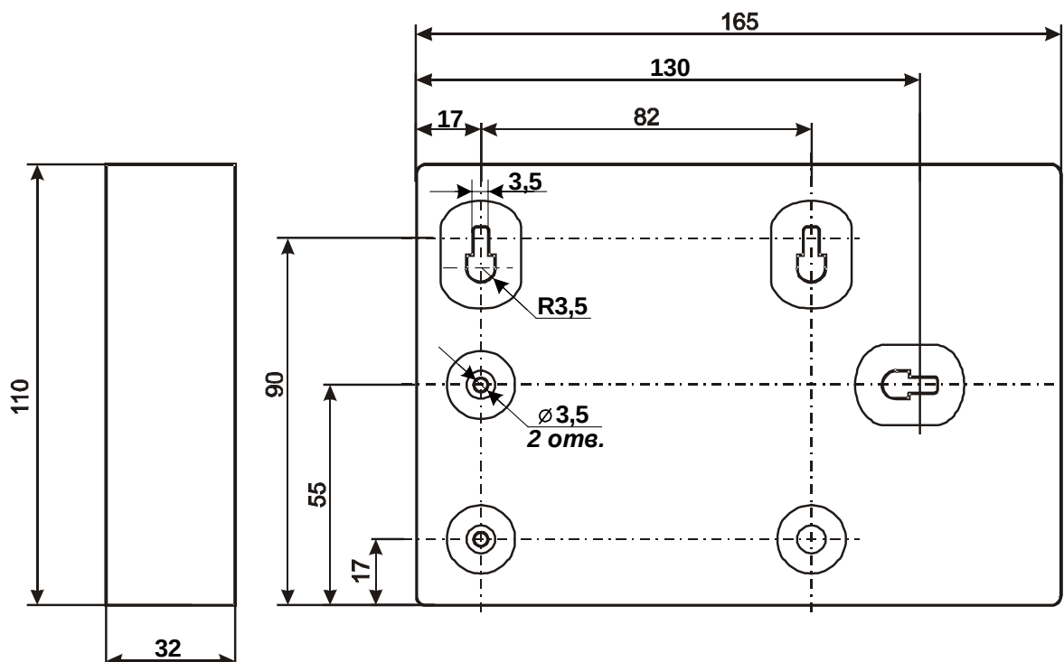
Рис. 3 Габаритные и присоединительные размеры БЦП исп. 7У.
