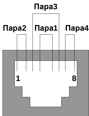
Рис. 7 Подключение ППК и ПЭВМ (Ethernet)
