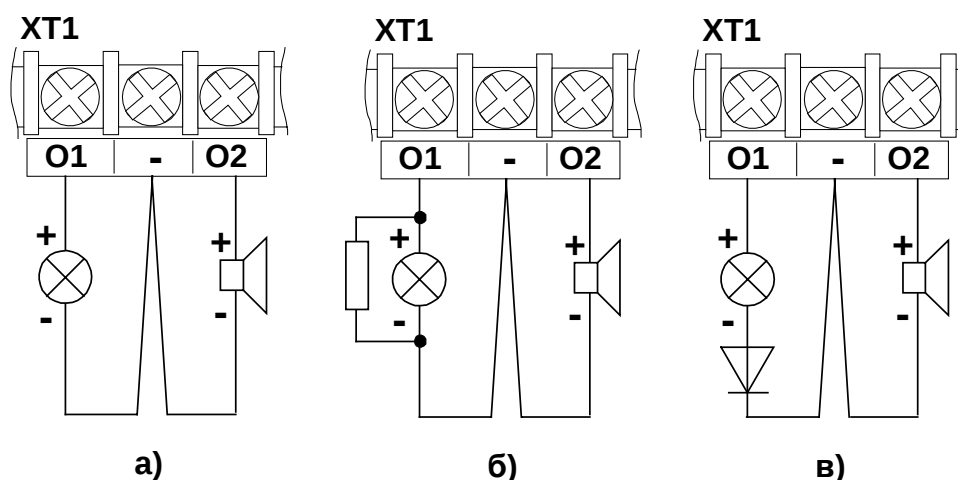
Рис. 9 Варианты подключения оповещателей
