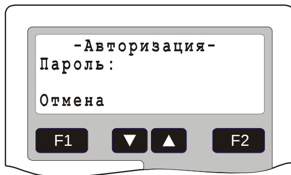
Рис. 2 Окно авторизации
