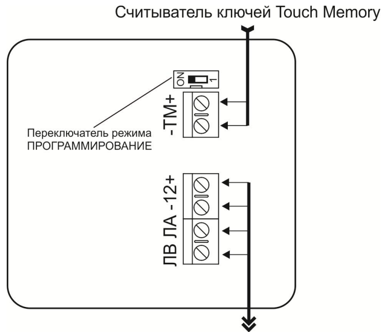
Рис. 4. Схема внешних соединений блока клавиатуры.
