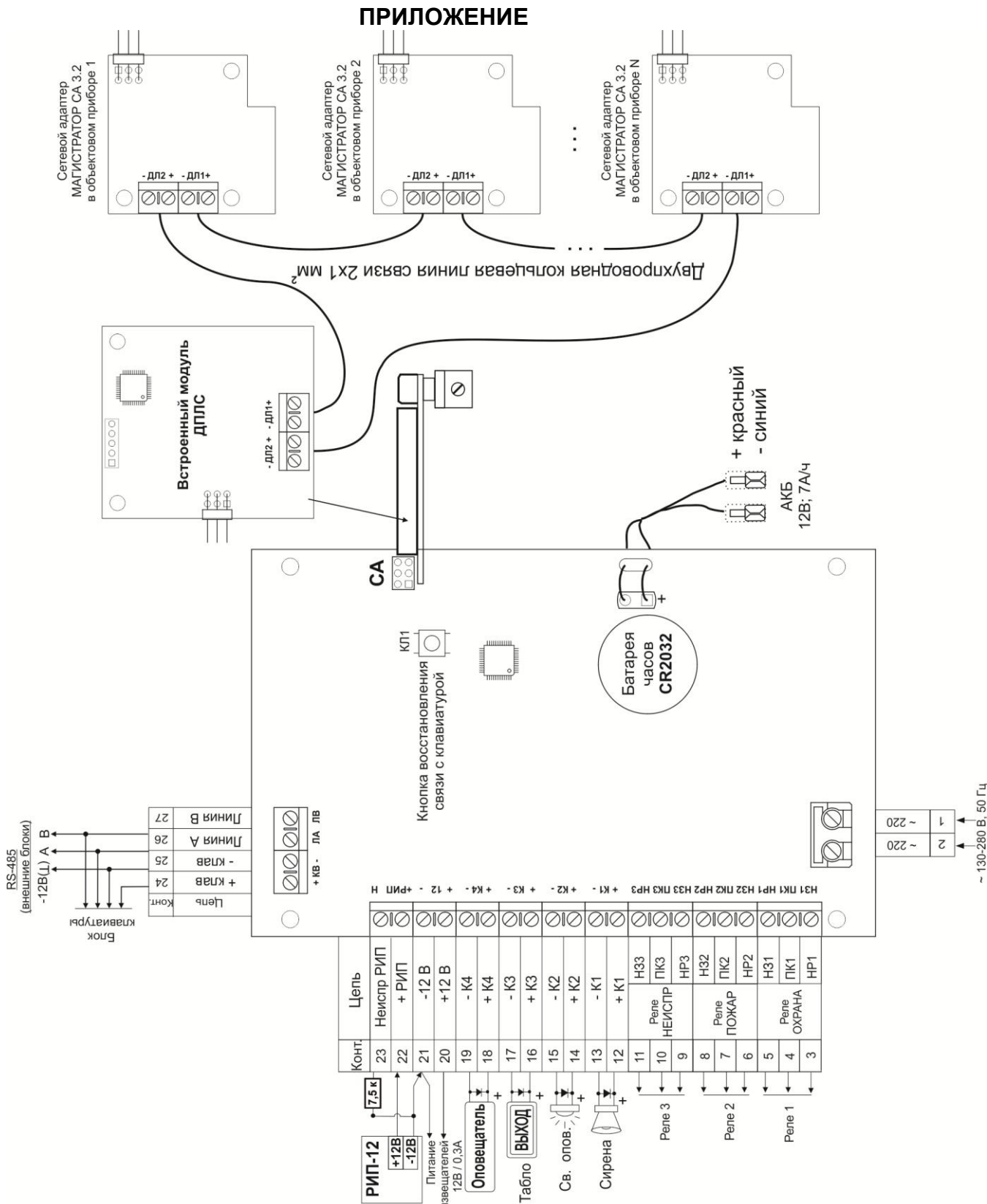
Рис. 3. Схема внешних соединений системного блока «МАГИСТРАТОР» (версия 3.2)
