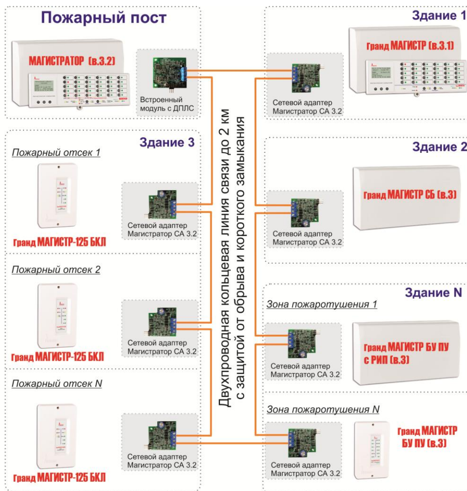
Рис 2. Принцип построения системы
