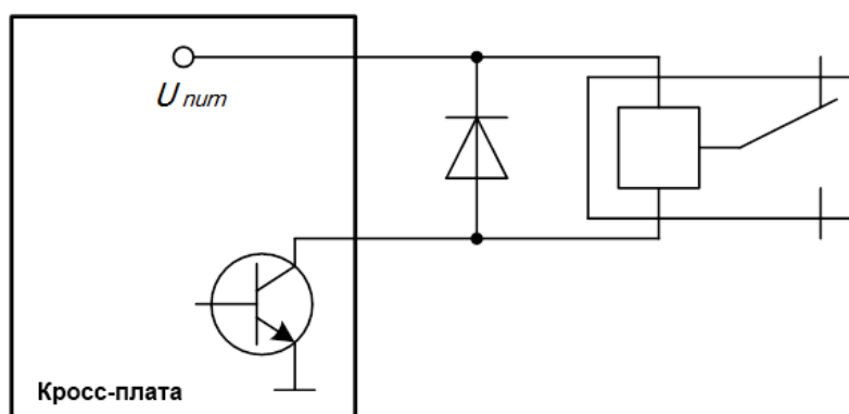
Рисунок 19 – Схема подключения диода параллельно обмотке реле
