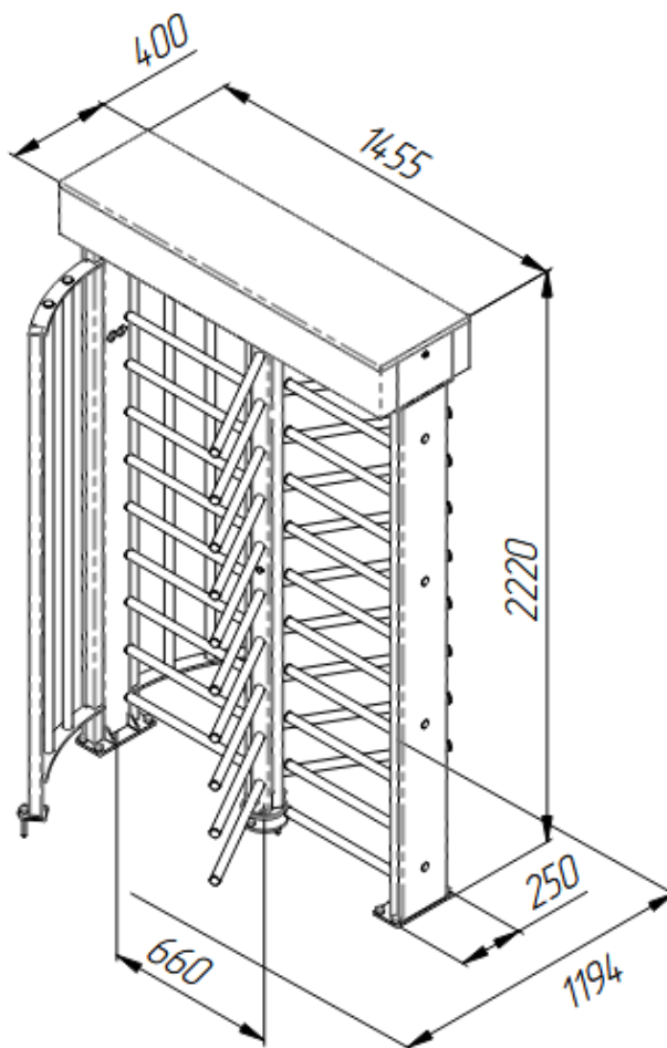
Рисунок 1 – Габаритные размеры турникета
