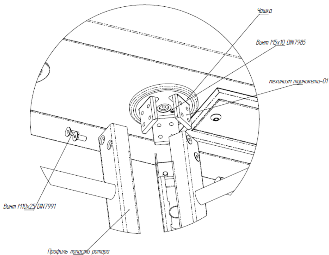
Рисунок 12 – Сборка роторной калитки (верх)
