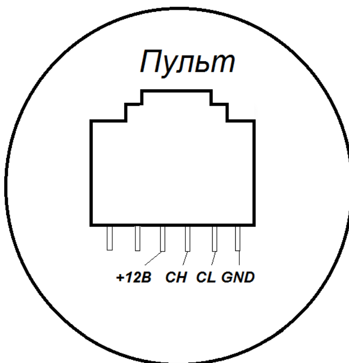
Рисунок 17 - Расположение проводов кабеля пульта управления.
