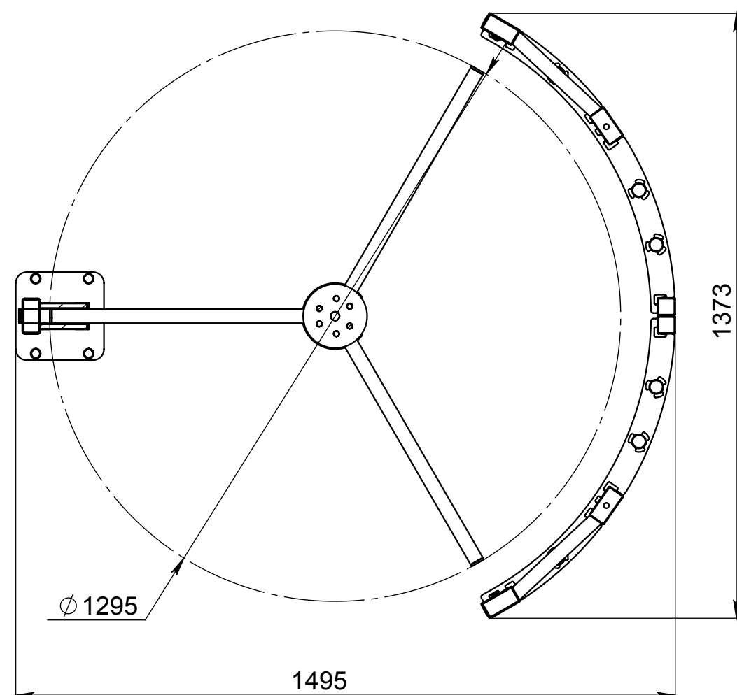
A-A (1 : 12)
