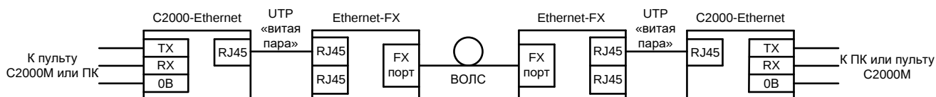
Рисунок 2.2.4 Схема подключения в режиме удлинения RS-232
