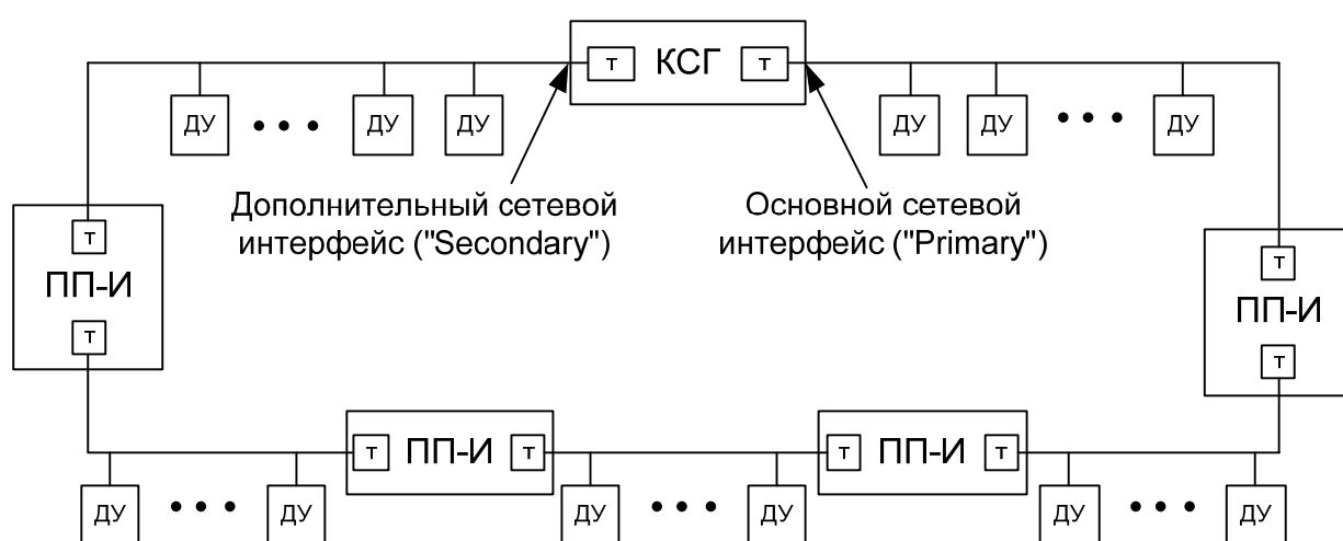
Рисунок 3 Кольцевая топология
