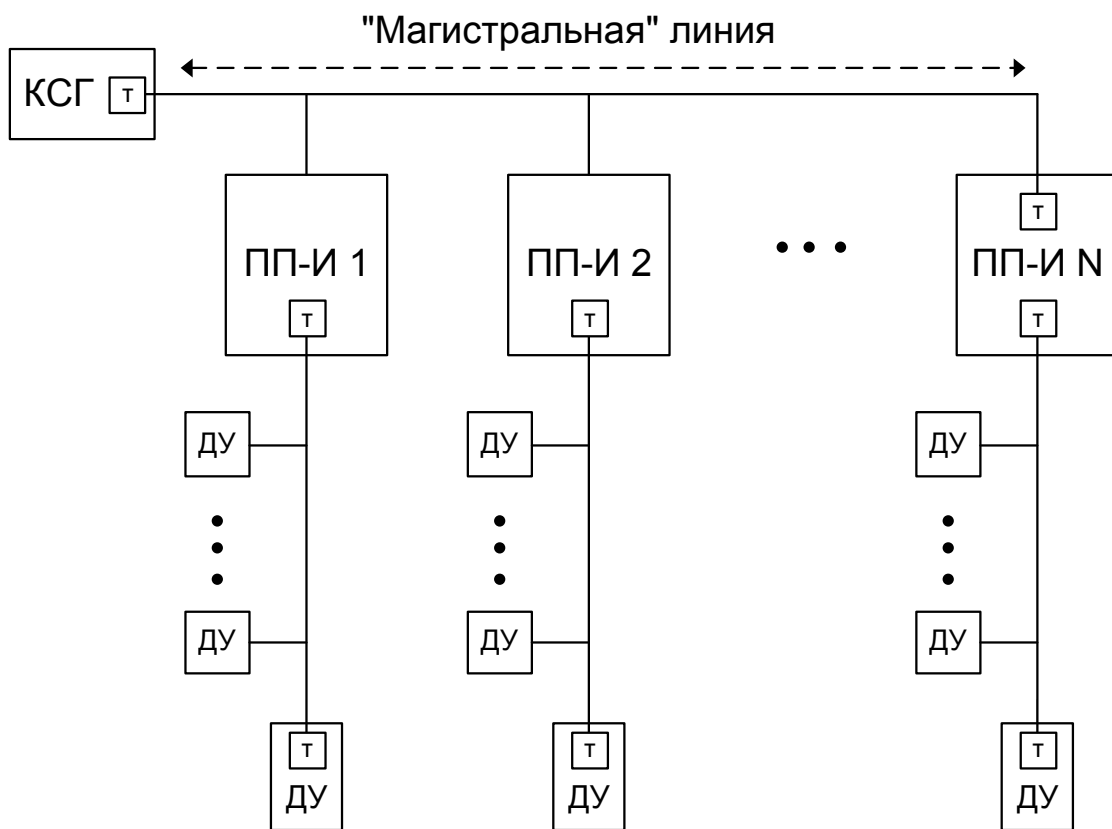
Рисунок 2 Радиальная топология
