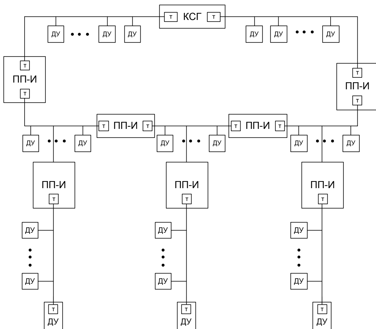
Рисунок 4 Пример построения свободной топологии
