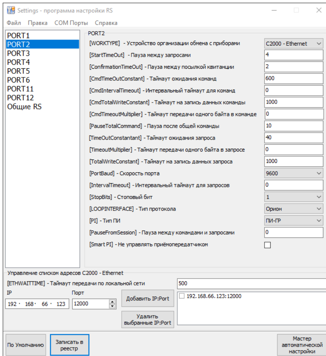
Рисунок 2.12. Утилита «Settings.exe»
