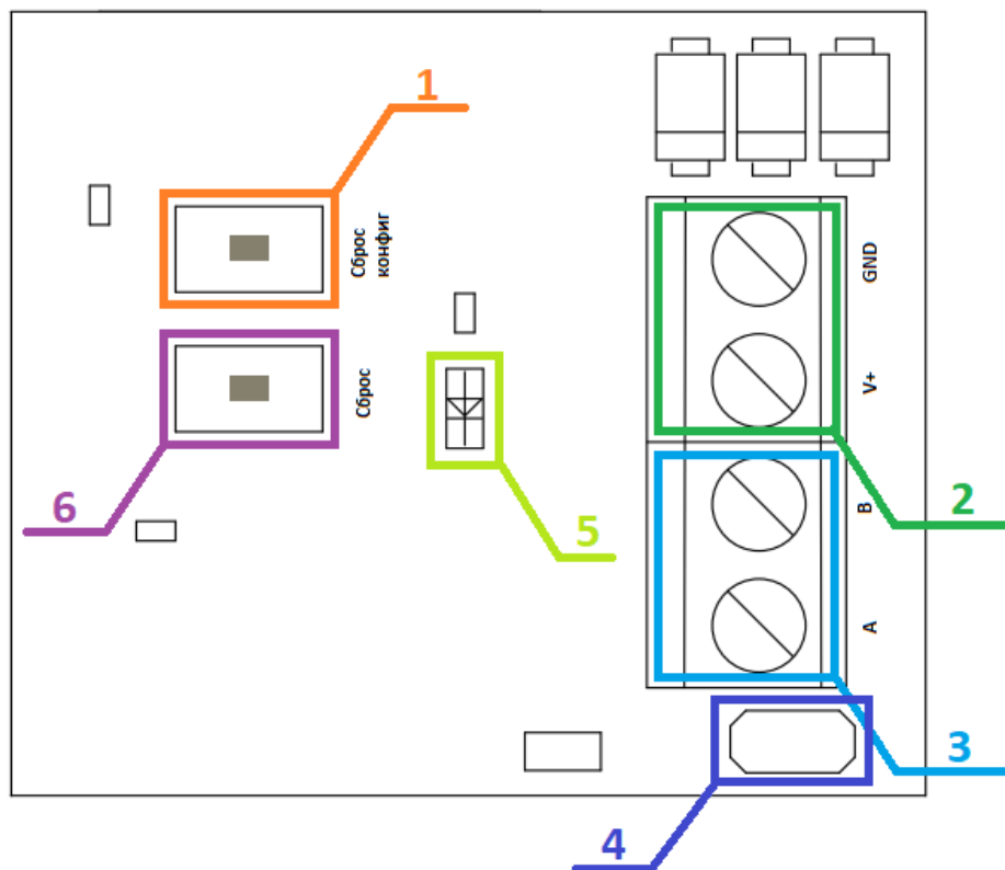
Рисунок 2.4. Расположение элементов прибора
