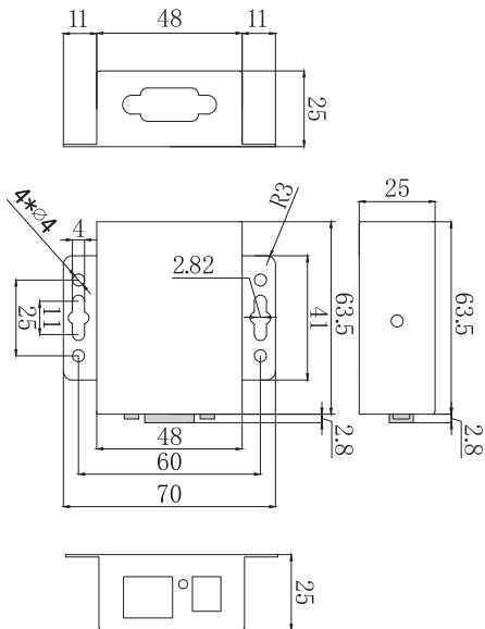
Рис.1 Габаритные размеры TSX-MC-232/485-TCP-MB
