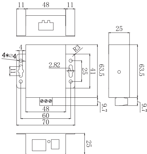
Рис.1 Габаритные размеры TSX-MC-485-TCP
