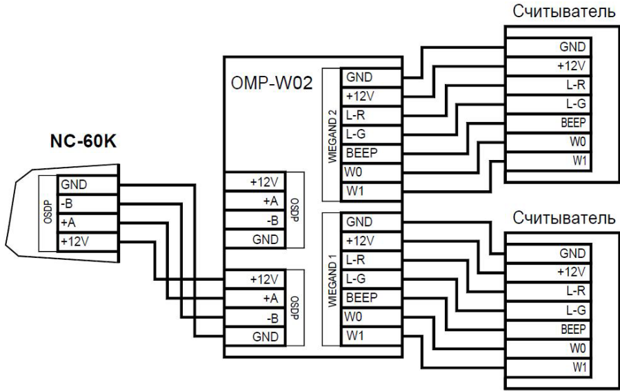
Рисунок 4. Подключение считывателей с питанием по шине OSDP
