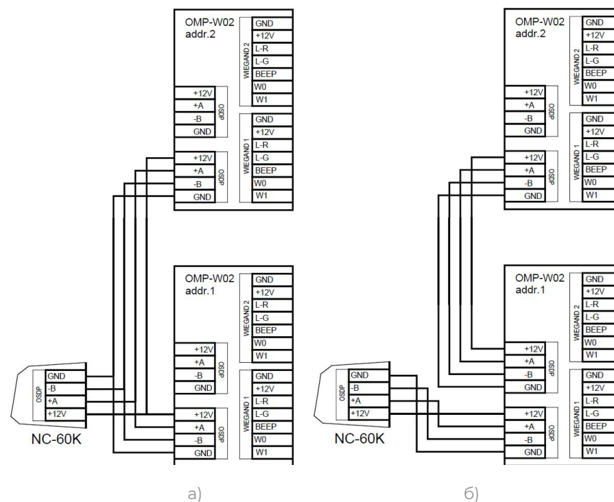
Рисунок 3. Схемы подключения преобразователей OMP-W02 к контроллеру
