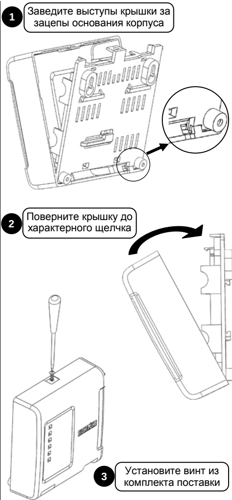
Рисунок 4. Установка крышки
