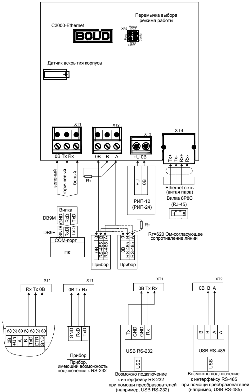
Рисунок 5. Схема внешних соединений преобразователя
