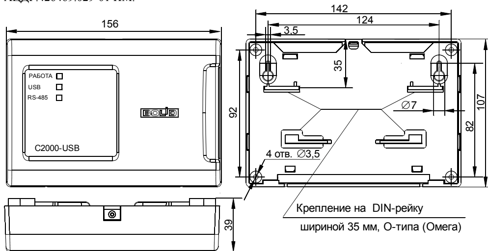
Рисунок 2. Габаритные и установочные размеры «C2000-USB»
