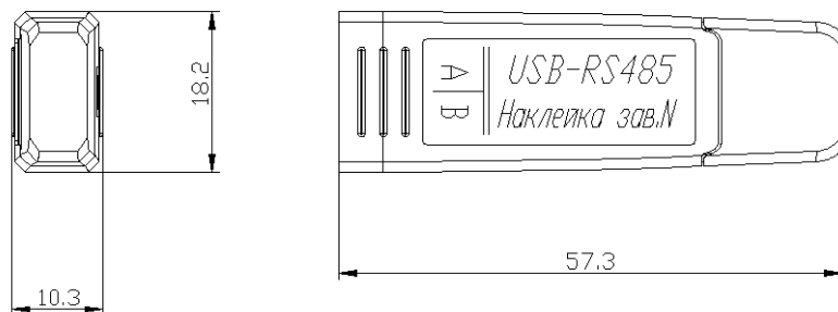
Рисунок 2. Габаритные размеры «USB-RS485»
