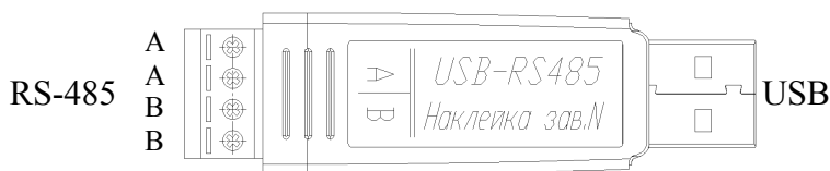
Рисунок 1. Схема подключения «USB-RS485»
