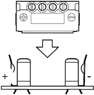
Рисунок 5 - Установка БП-3В в разъем CR123A
