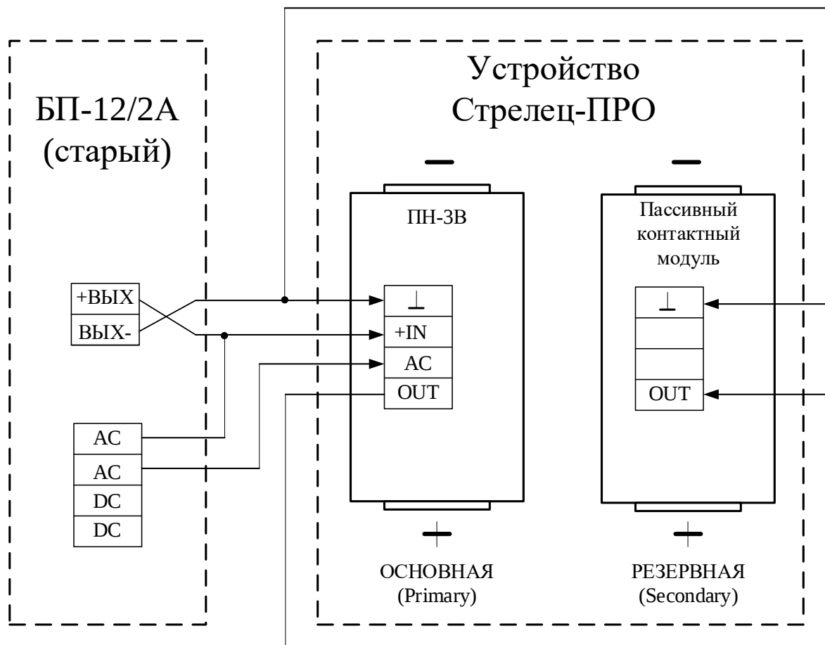
Рисунок 3 - Подключение ПИ-3В с контролем внешнего источника питания
