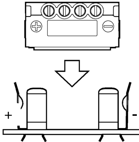
Рисунок 5 - Установка ПН-3В в разъем CR123A
