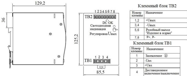
Габаритные размеры изделия и назначение клемм
