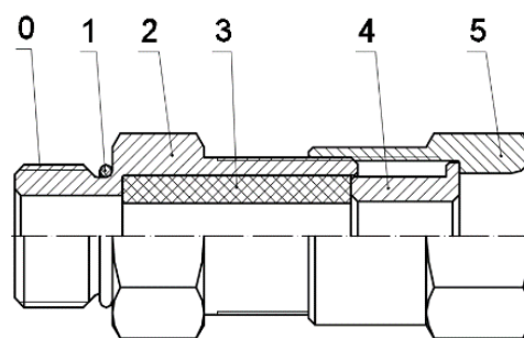
КВН – для монтажа открытого кабеля
