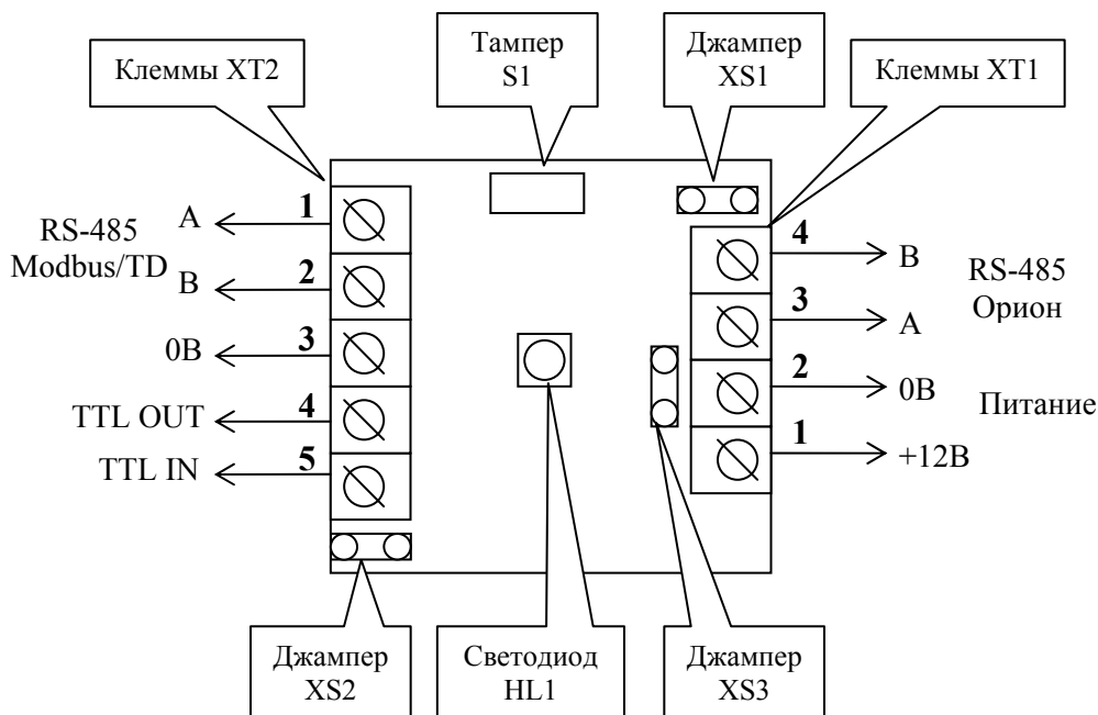
Рис. 3. Плата «С2000-ПП»
