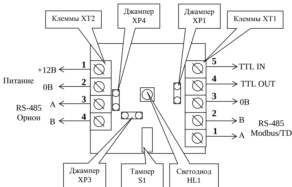
Рисунок 1. Плата «С2000–ПП» версии 3.xx
