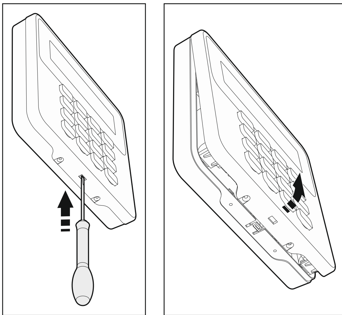
Рис. 2. Открытие корпуса.
