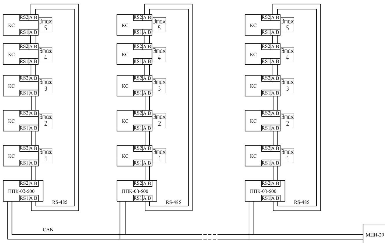
Рисунок 7 – Схема организации интерфейса RS-485
