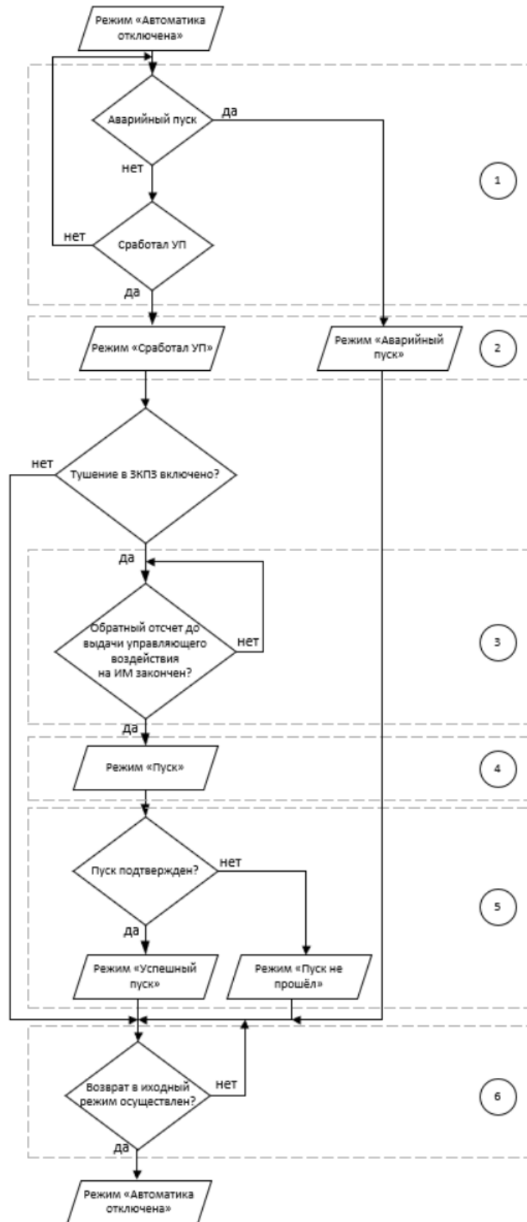
Рисунок 4.2 – Алгоритм фиксации режимов «Аварийный пуск», «Пуск (выдача сигнала на ИМ противопожарной защиты)», «Сработал УП» в режиме «Автоматика отключена» ЗКПЗ
