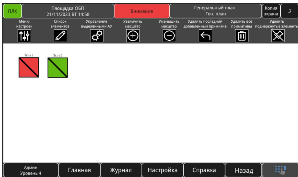
Рисунок 3.120 – элементы-ЗКПЗ
