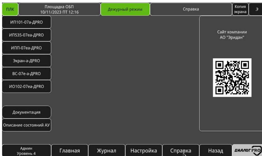
Рисунок 3.141 – Окно «Справка»
