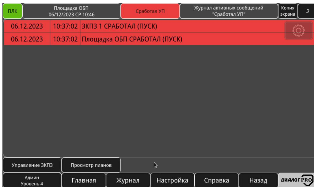
Рисунок 3.28 – Окно «Журнал активных сообщений «Сработал УП»
