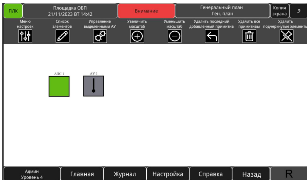
Рисунок 3.118 – элементы-АУ
