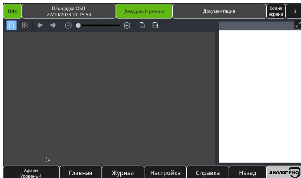
Рисунок 3.144 – Окно «Документация»
