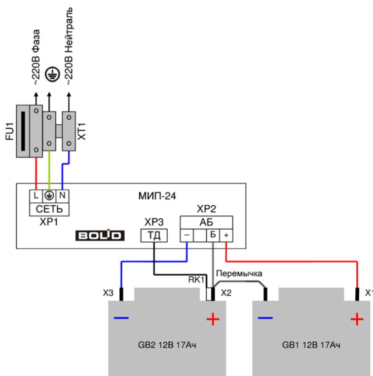
Рисунок 68. Схема подключения источников питания
