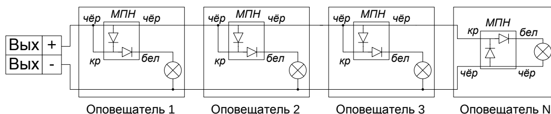
Рисунок 63. Схема подключения нескольких сирен или световых табло
