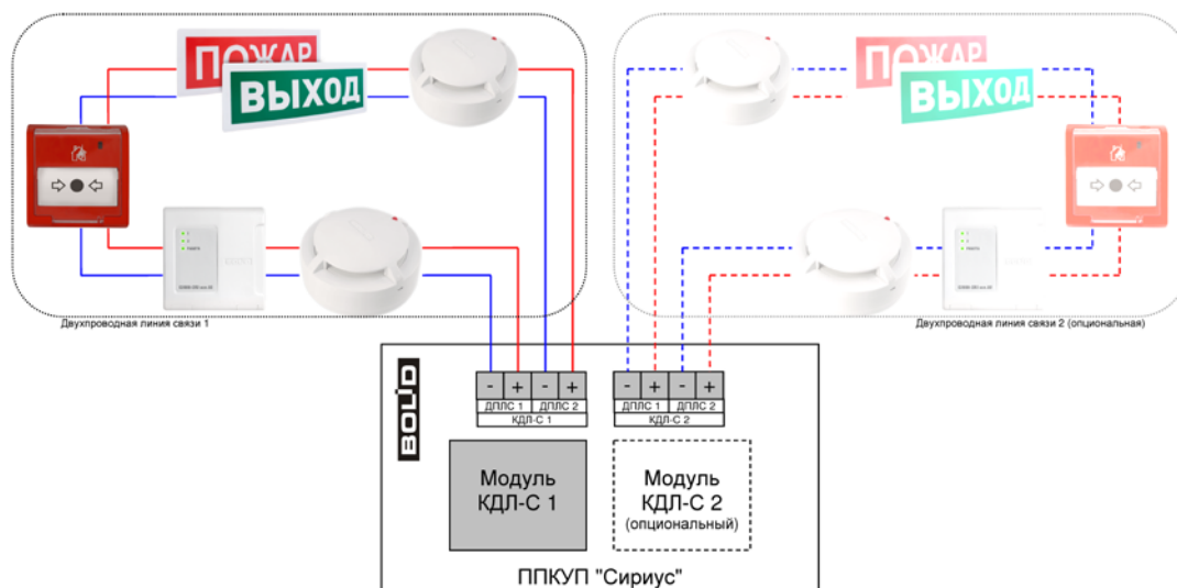
Рисунок 60. Схема подключения адресных устройств
