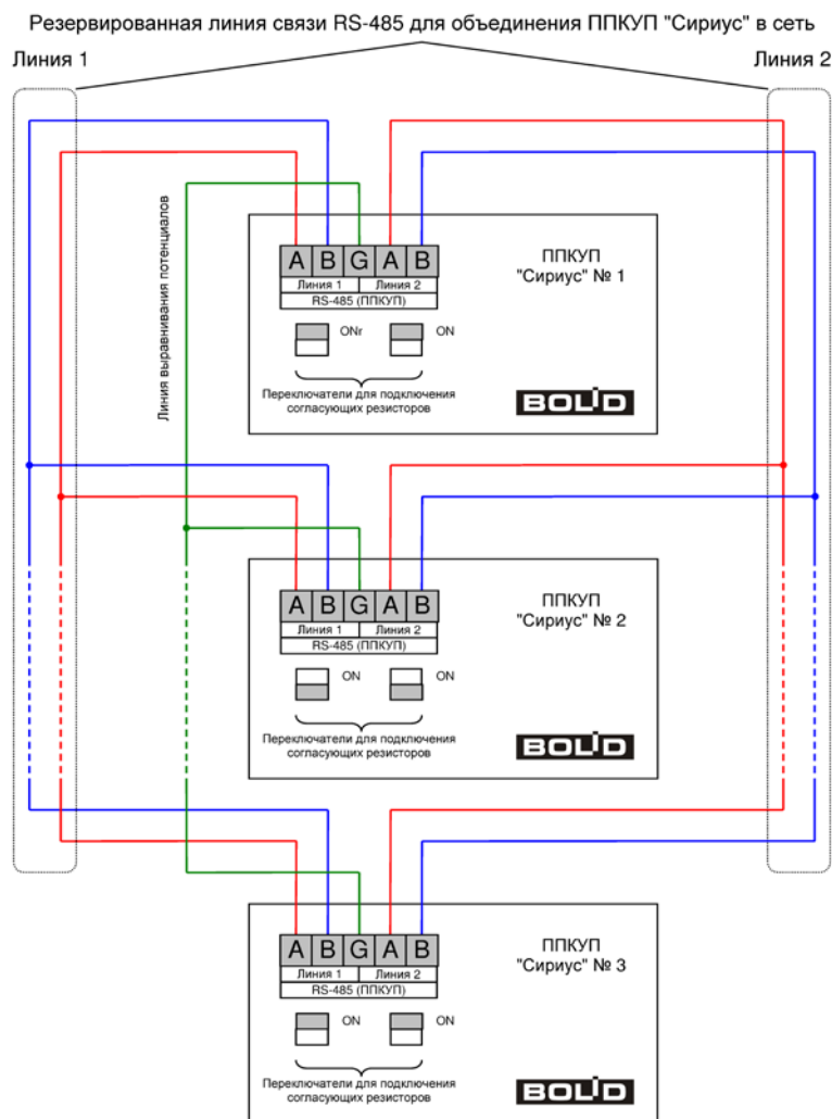
Рисунок 67. Схема объединения приборов «Сириус» в сеть
