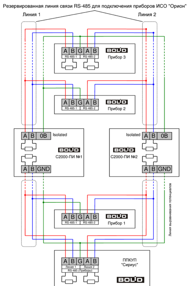
Рисунок 65. Схема подключения повторителей резервированного интерфейса RS-485 «С2000-ПИ»
