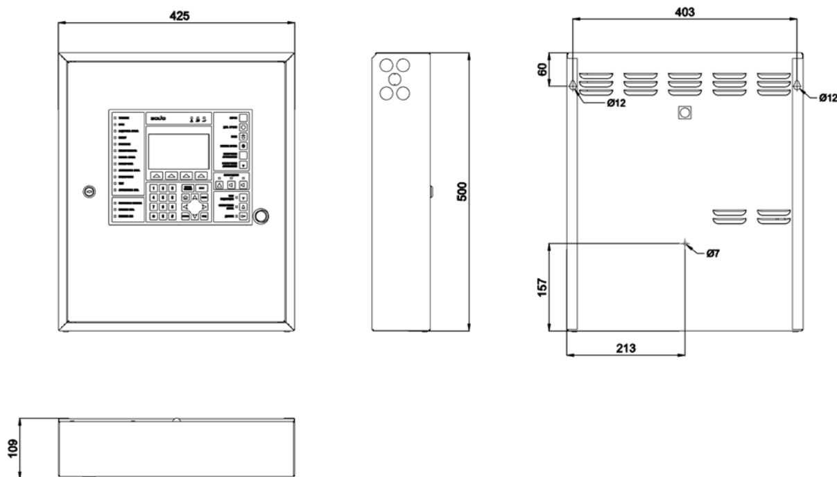
Рисунок 59. Габаритные и установочные размеры
