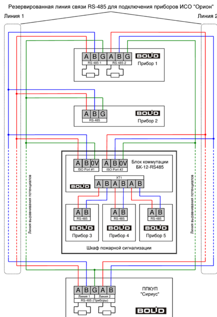
Рисунок 64. Схема подключения дополнительных блоков и приборов ИСО «Орион»
