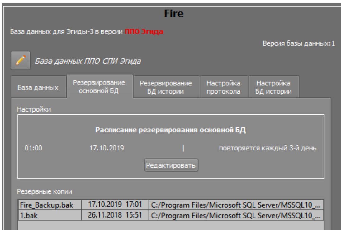
Рисунок 4-37. Вторая вкладка конфигуриатора БД – «Резервирование основной БД»
