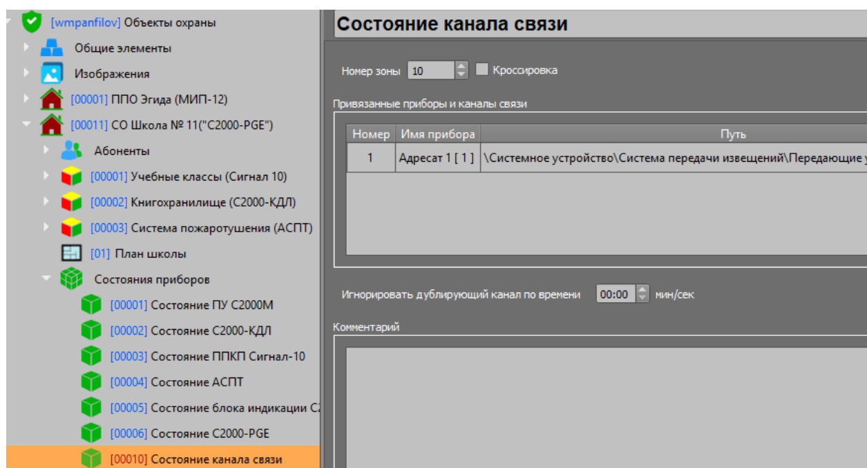
Рисунок 3-98. Настроенная зона состояния адресата «C2000-PGE»
