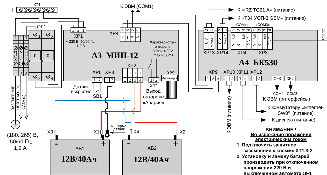
Рисунок 2-3. Схема подключения питания в ППО КСПИ Эгида
