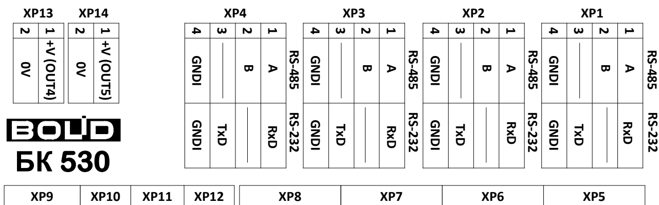
Рисунок 2-4. Схема подключения интерфейсов RS232 к ППО КСПИ Эгида
