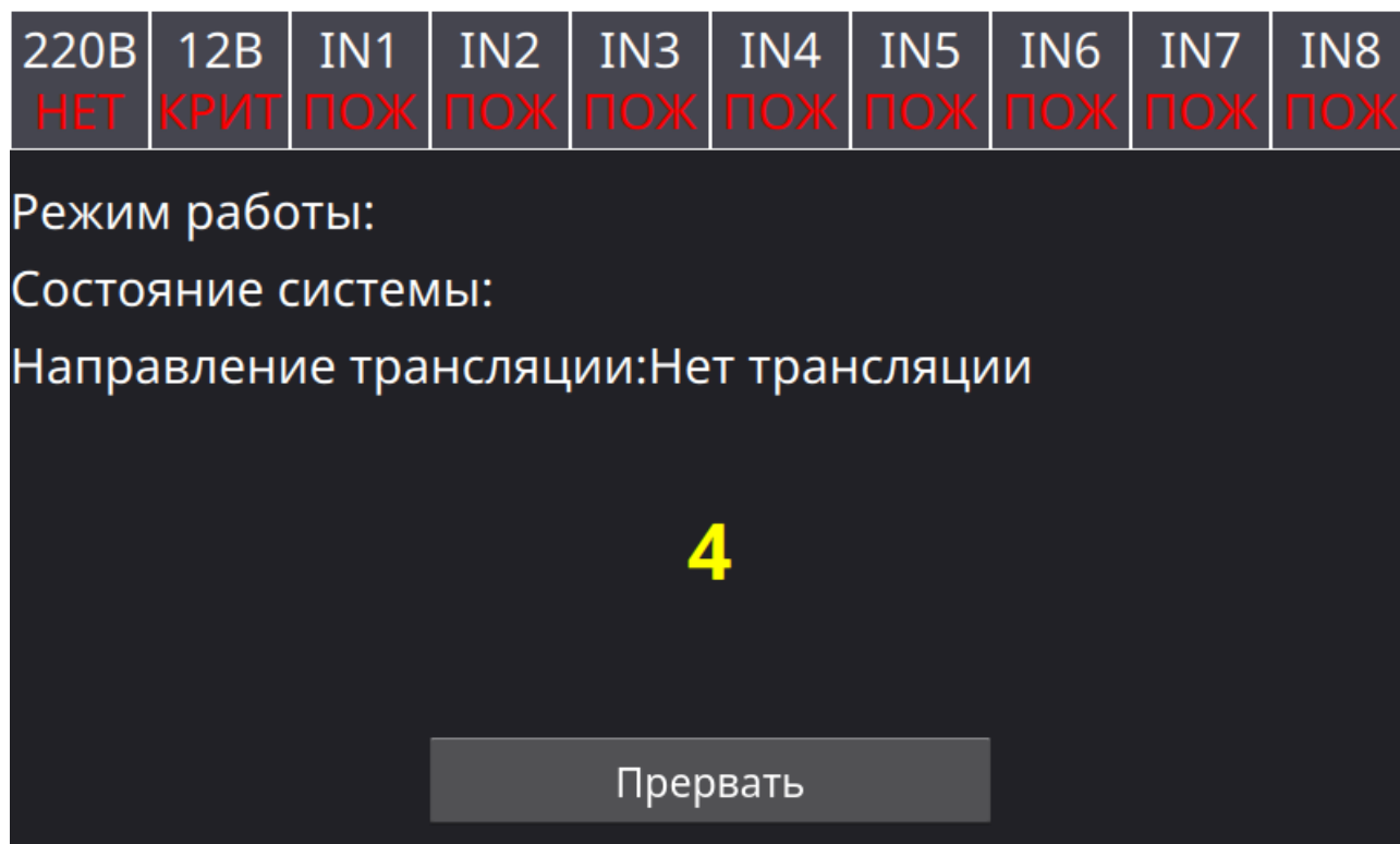
Рисунок 40 - Раздел «Тест».
