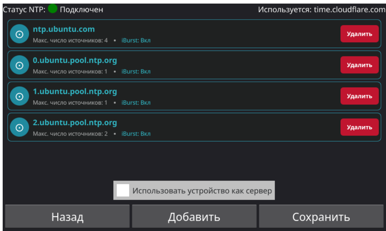
Рисунок 27 - NTP сервер
