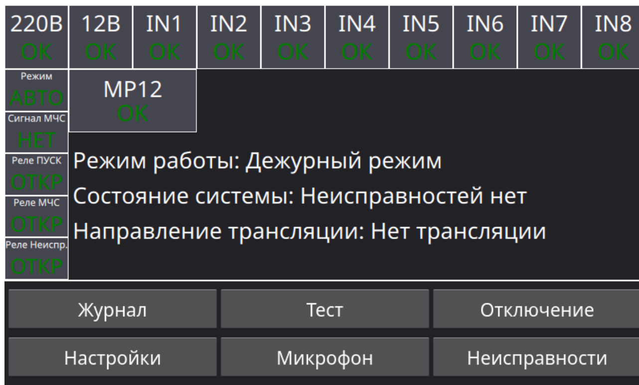
Рисунок 10 - Дежурный режим
