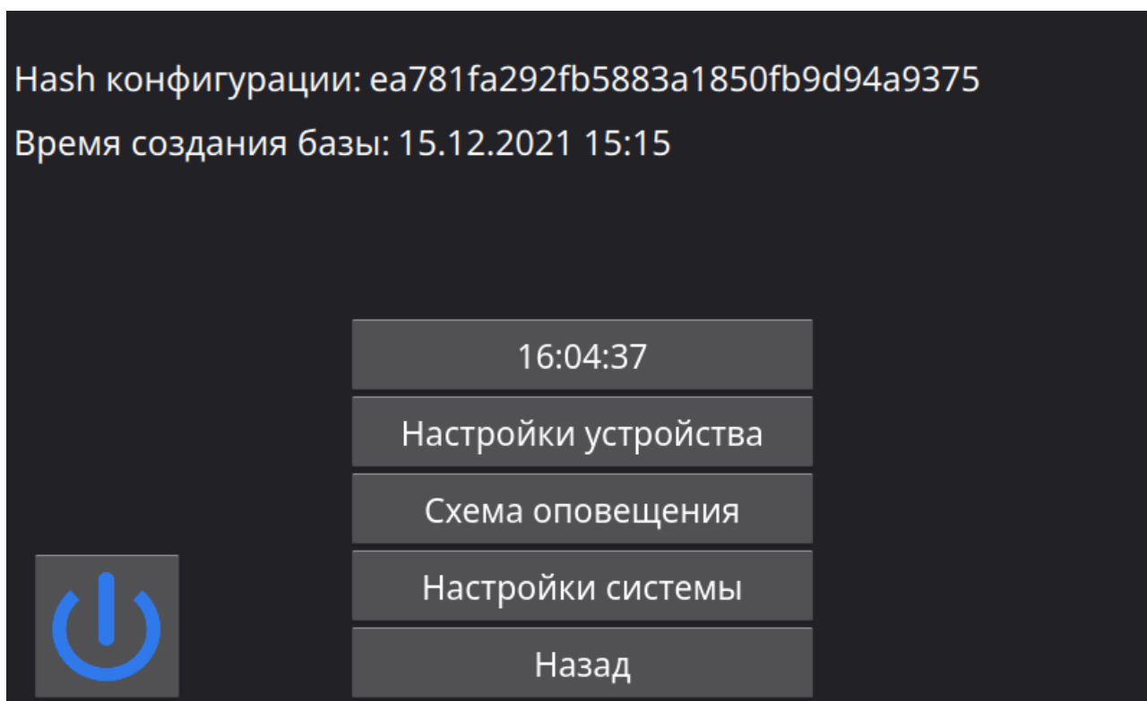
Рисунок 25 - Раздел «Настройки»
