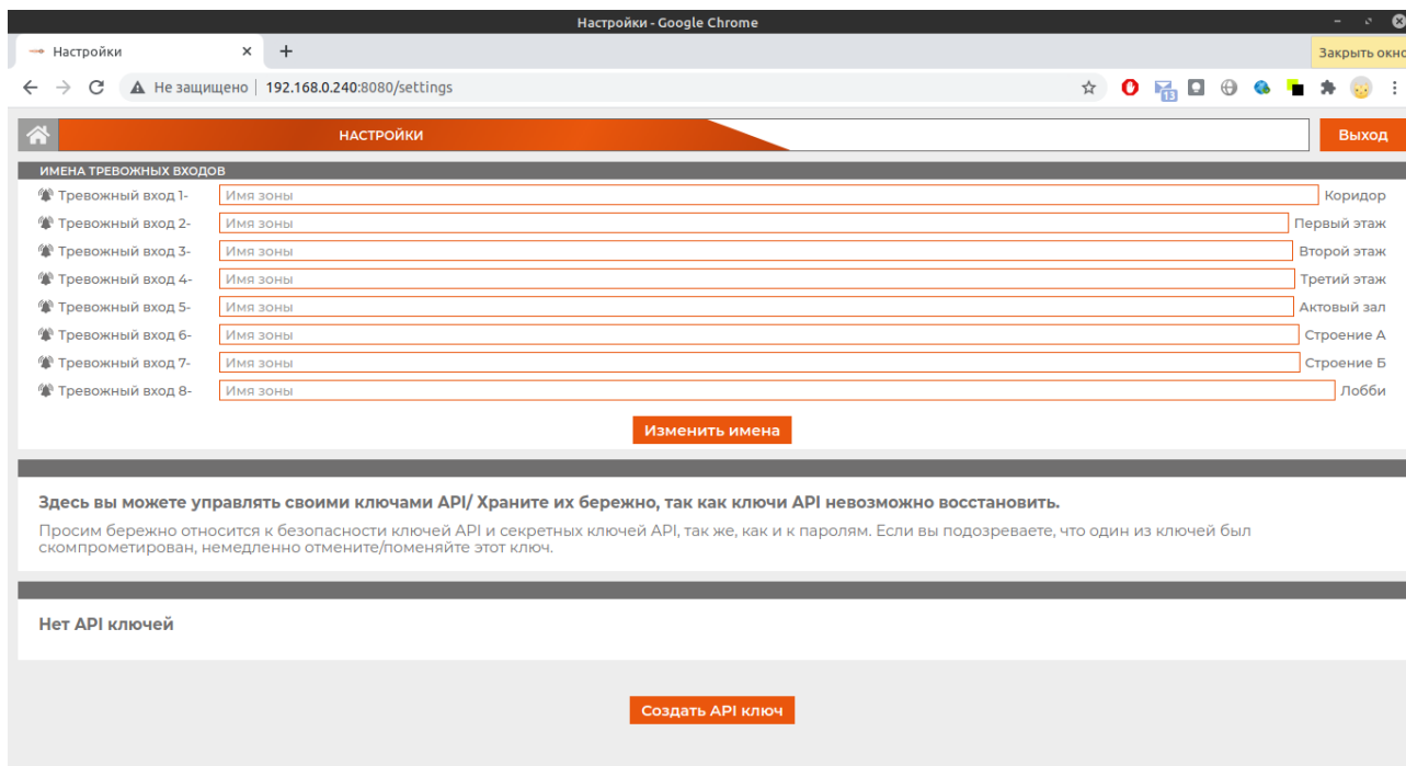
Рисунок 47 - Имена зон
