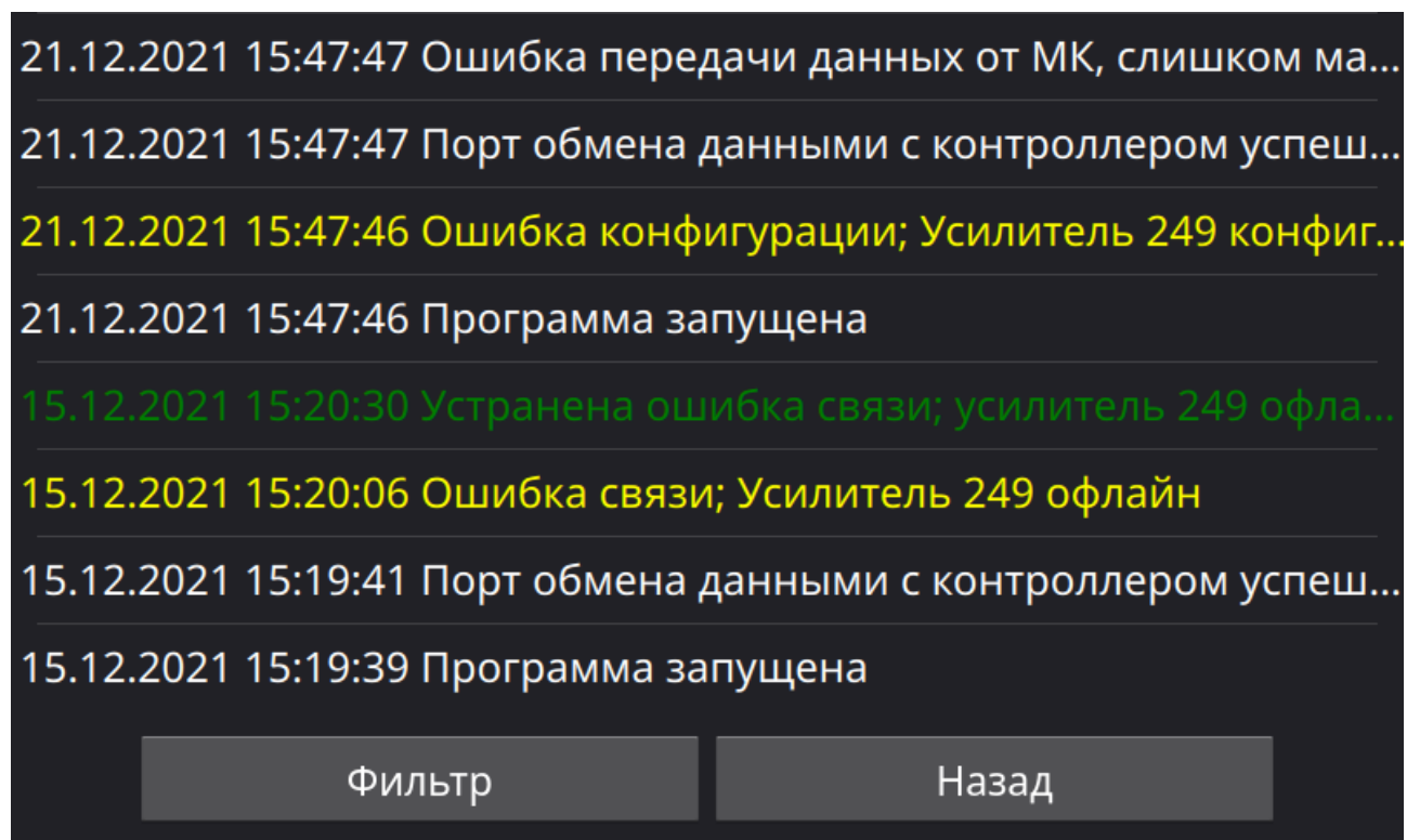
Рисунок 35 - Раздел «Журнал»
