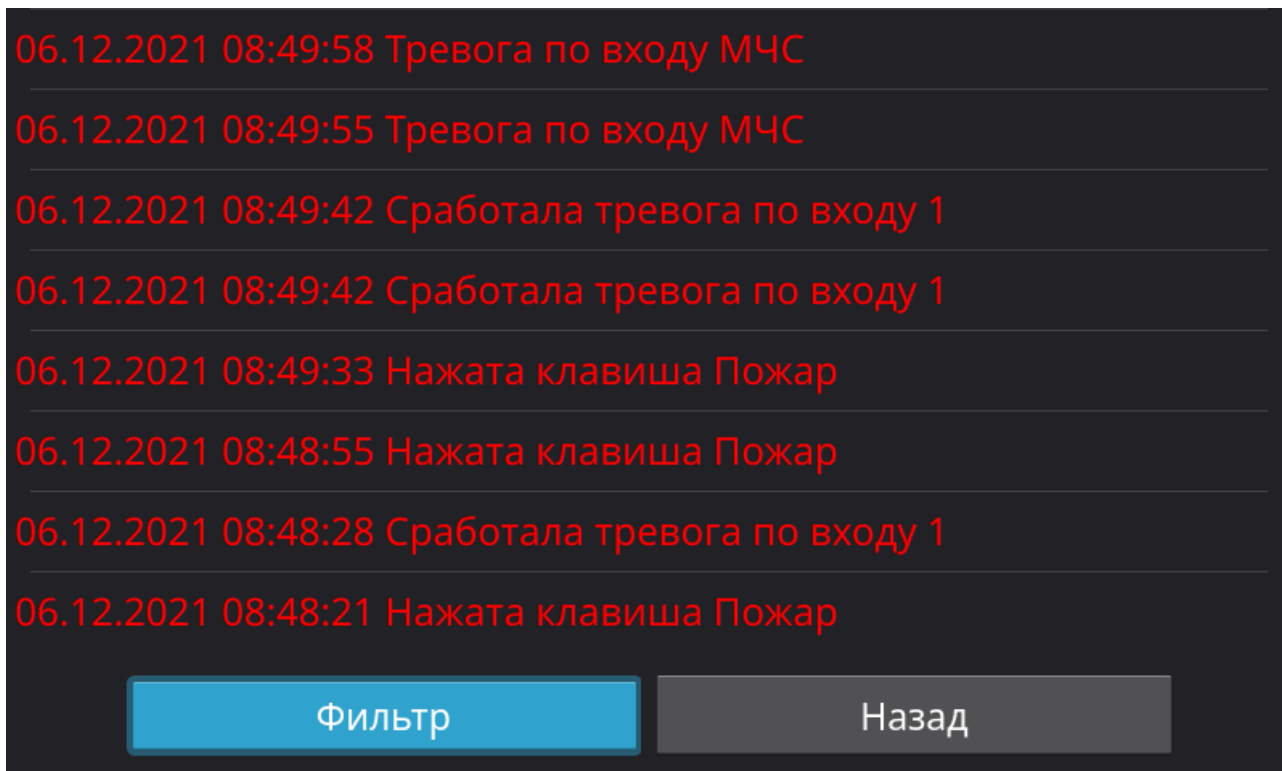
Рисунок 39 - Отфильтрованные события
