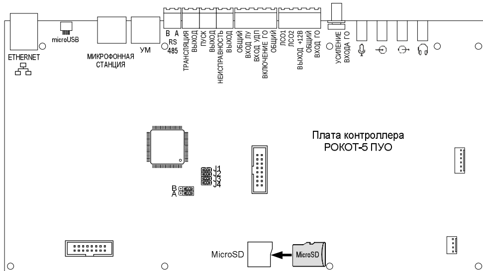
Рисунок А6 – Внешний вид платы контроллера ПУО (интерфейс «RS-485 АВ» в данной версии ПУО не используется)
