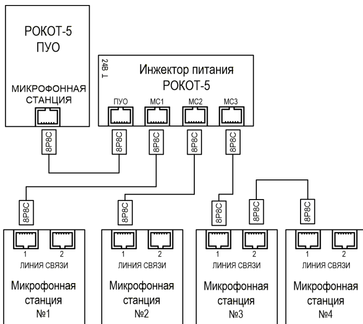
Рисунок А9 – Схема подключения микрофонных станций MC-2 к «РОКОТ-5 ПУО» через инжектор питания
