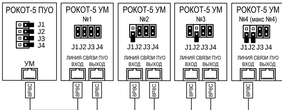
Рис.А5 Схема подключения усилителей «РОКОТ-5 УМ» к «РОКОТ-5 ПУО» (всего можно подключить до 4-х усилителей мощности).
