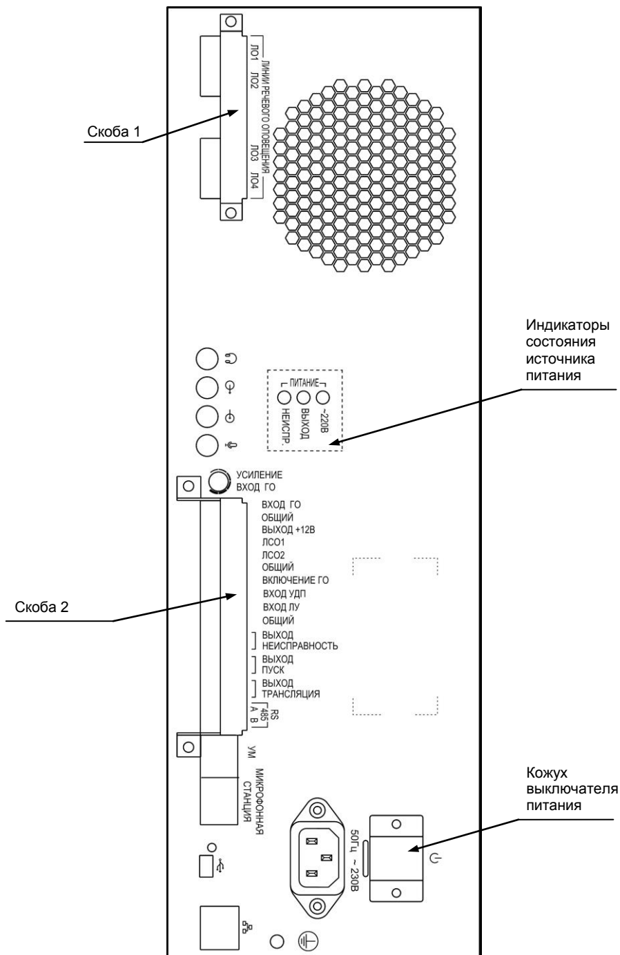
Рис.2 Внешний вид задней панели
