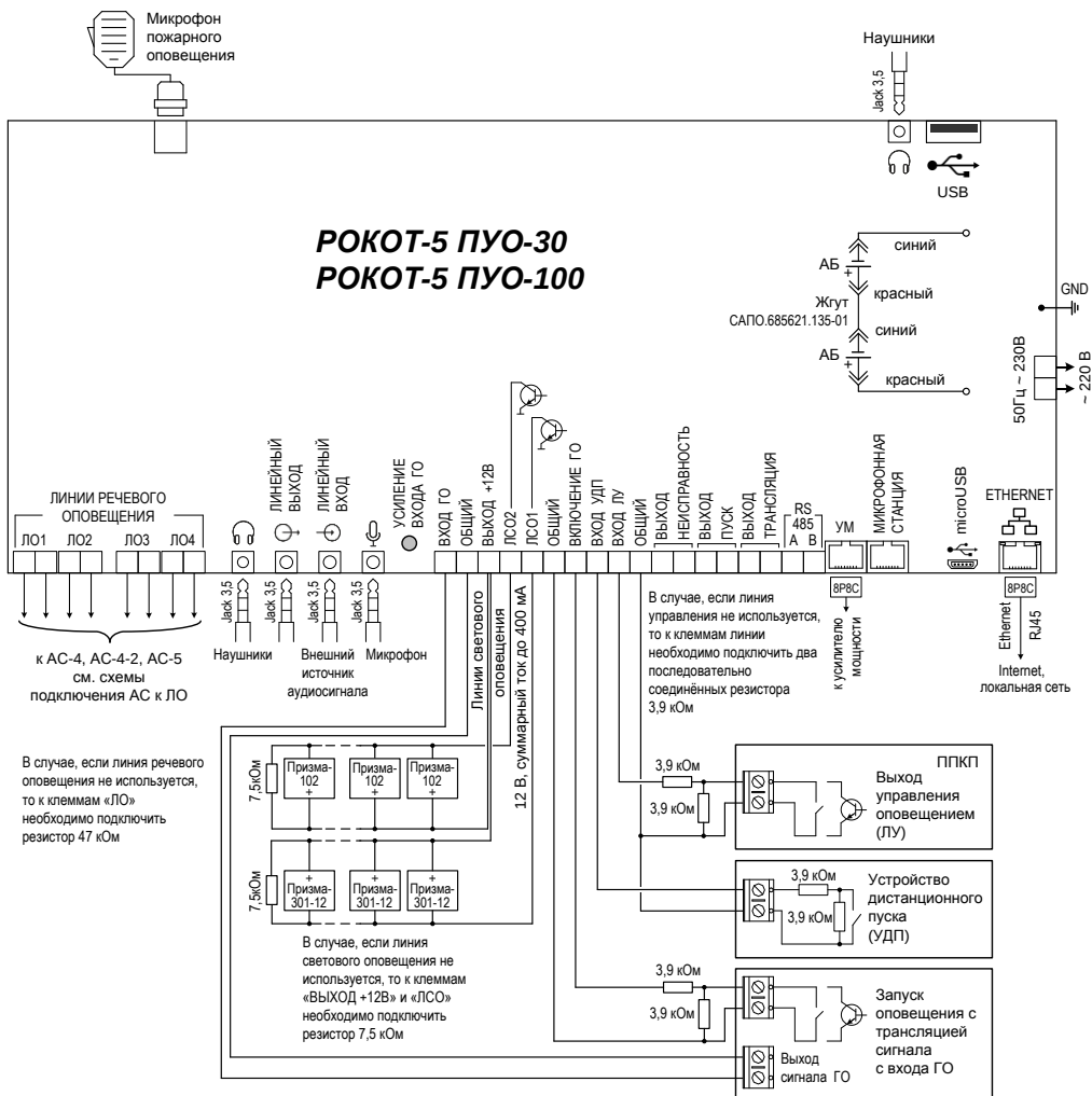
Рис.А1 Схема внешних подключений «РОКОТ-5 ПУО» (интерфейс RS-485 в данной версии ПУО не используется)
