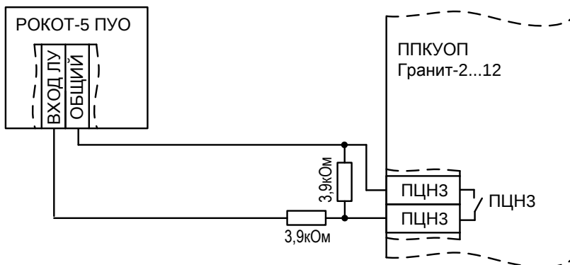
Рис.А2 Схема подключения ПУО к ППКУОП «Гранит-2,-3,-4,-5,-8,-12,-16,-20,-24»
