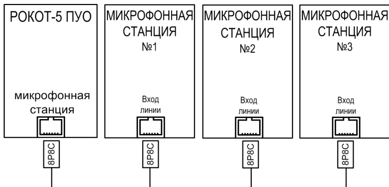
Рис.А8 Схема подключений микрофонных станций к «РОКОТ-5 ПУО» (всего можно подключить до 3-х микрофонных станций).
