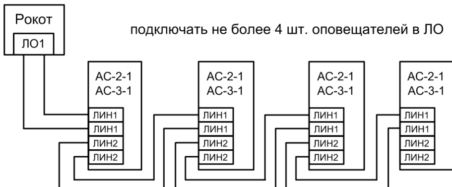
Рис.А3 Схема подключения оповещателей «AC-2-1», «AC-3-1» (параллельное соединение)
