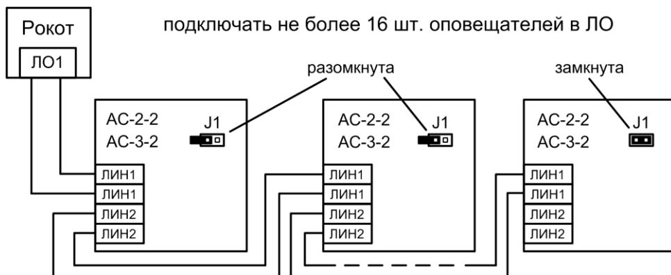
Рис.А5 Схема подключения оповещателей «AC-2-2», «AC-3-2» (параллельное соединение)
