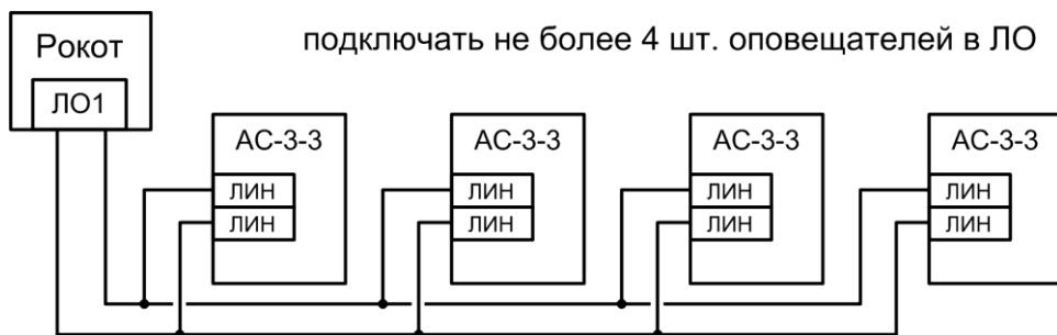
Рис.А4 Схема подключения оповещателей «AC-3-3» (параллельное соединение)
