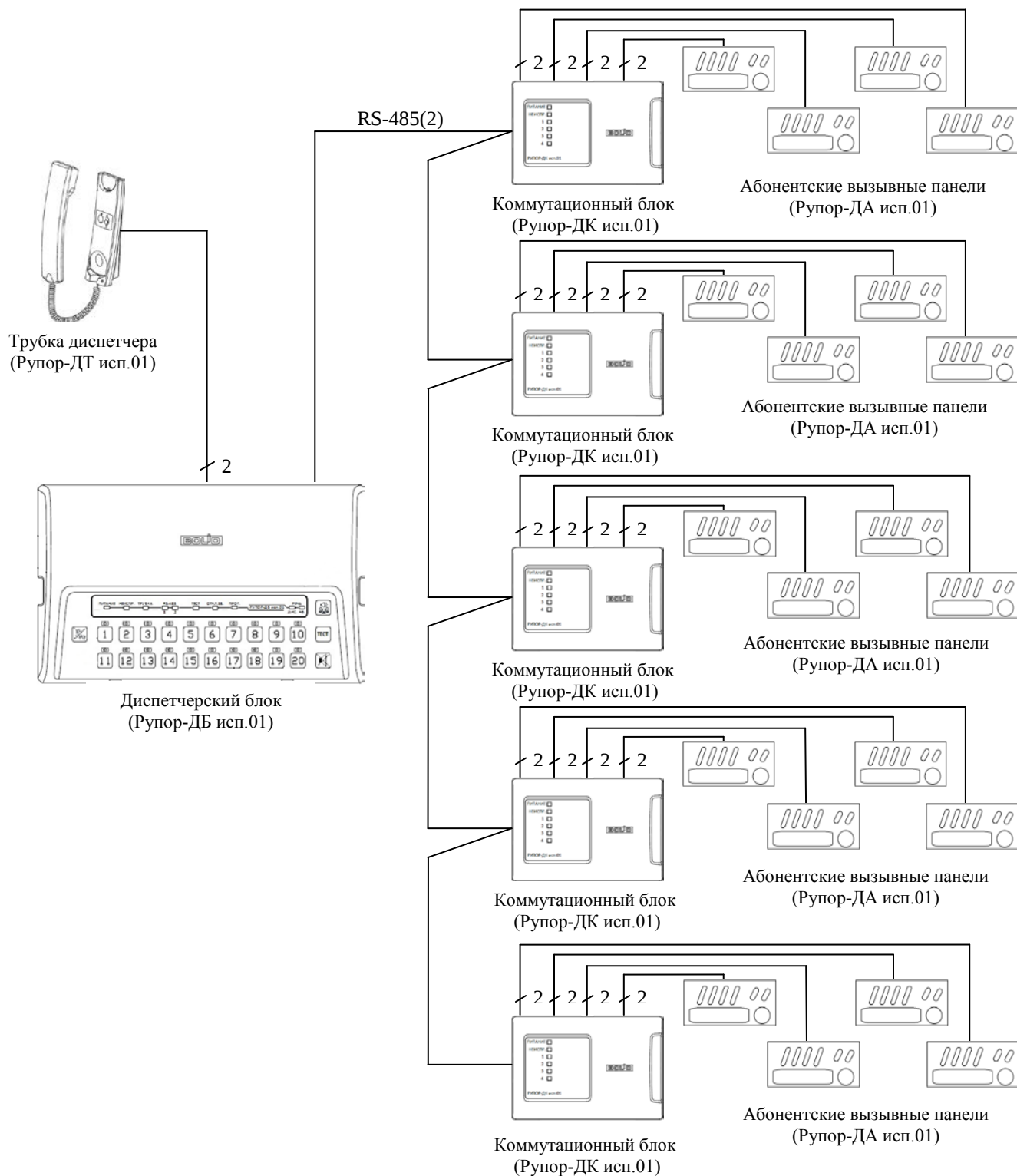
Рисунок 1.3.1 – Подключение блоков при автономном использовании комплекса.
