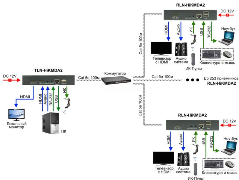
Рис.9 Схема подключения комплекта TLN-HiKMDA2+RLN-HiKMDA2 через коммутатор в режиме «точка-многоточка»
