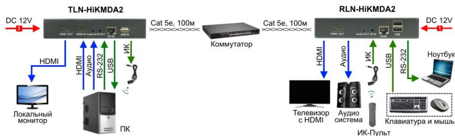
Рис.8 Схема подключения комплекта TLN-HiKMDA2+RLN-HiKMDA2 в режиме «точка-точка» через коммутатор
