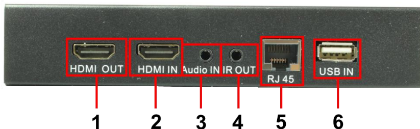
Рис.3 Передатчик TLN-HiKMDA2, разъемы и индикаторы на задней панели
