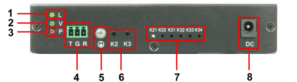
Рис.4 Приемник RLN-HiKMDA2, разъемы и индикаторы на передней панели
