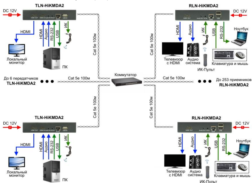
Рис.10 Схема подключения комплекта TLN-HiKMDA2+RLN-HiKMDA2 через коммутатор в режиме «многоточка-многоточка»
