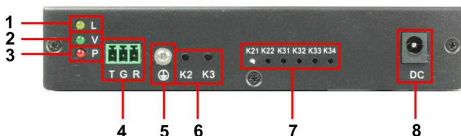
Рис.2 Передатчик TLN-HiKMDA2, разъемы и индикаторы на передней панели
