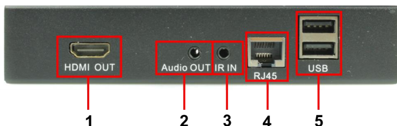
Рис.5 Приемник RLN-HiKMDA2, разъемы и индикаторы на задней панели
