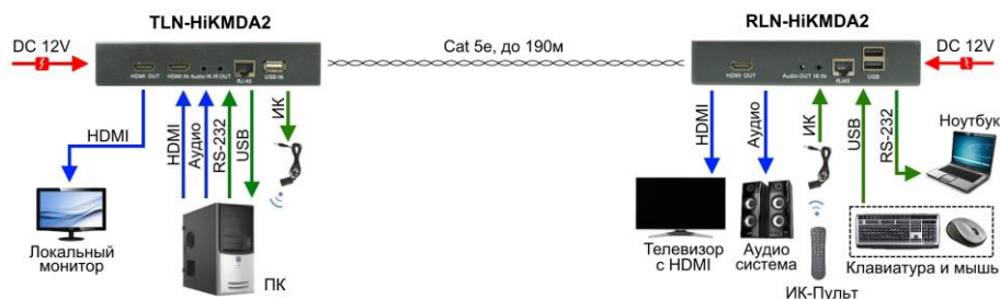
Рис.7 Схема подключения комплекта TLN-HiKMDA2+RLN-HiKMDA2 в режиме «точка-точка»
